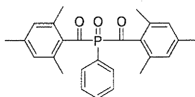
IRGACURE 819
