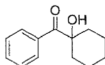
IRGACURE 184
