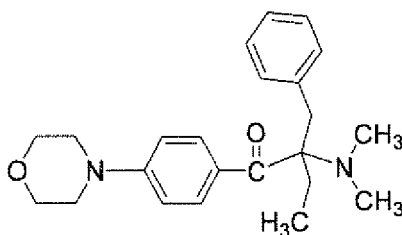
IRGACURE 369
