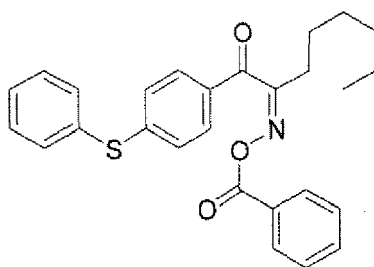
IRGACURE OXE-01
