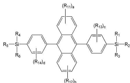
<화학식 1C>
