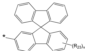
화학식 4D
