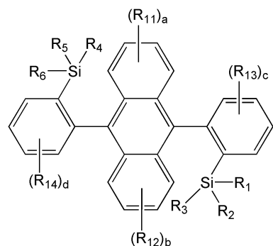
<화학식 1E>
