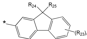
화학식 4C
