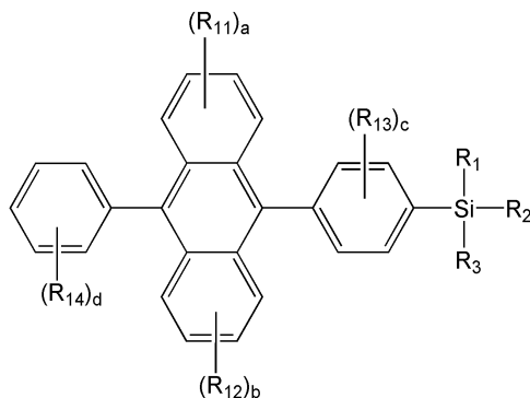
<화학식 1F>
