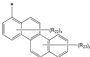
화학식 4I
