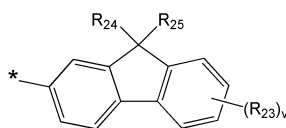
화학식 4C
