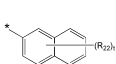
화학식 4A
