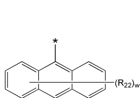
화학식 4G
