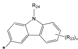
화학식 4E
