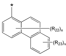
화학식 4H
