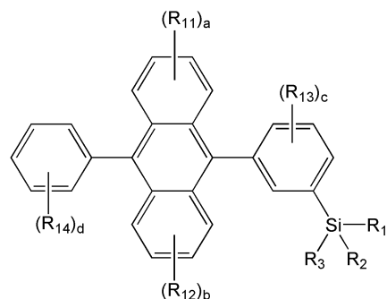
<화학식 1E>
