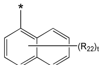
화학식 4B
