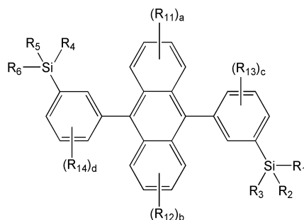
<화학식 1D>
