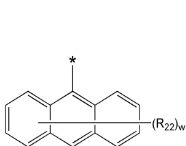
화학식 4G
