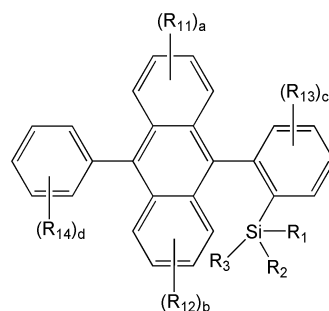
<화학식 1F>
