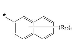
화학식 4A
