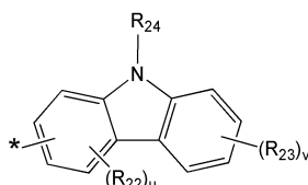
화학식 3E
