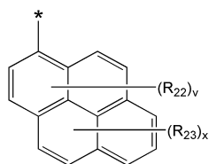
화학식 4J
