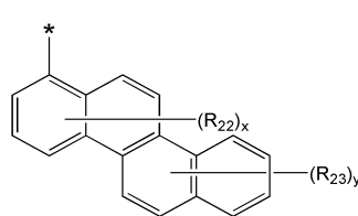
화학식 4I
