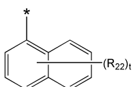
화학식 4B
