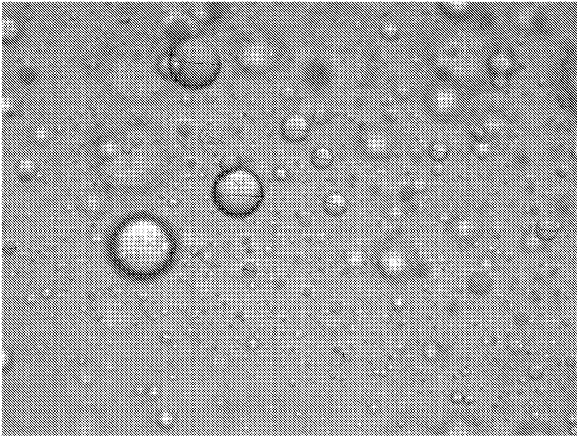
图1:在光学显微镜下采集的表5中1号试样的微观结构
