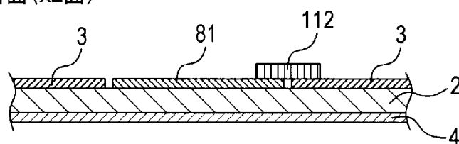
(b) C-C断面(xz面)
