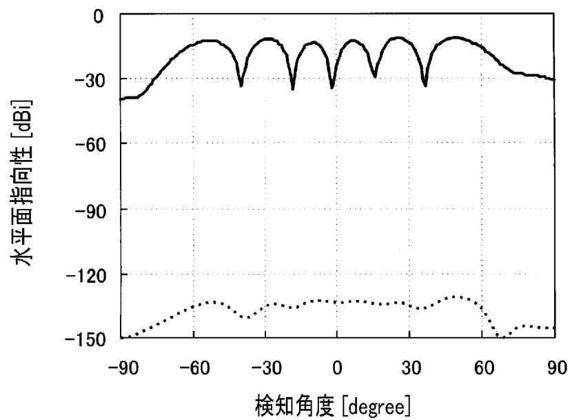
(b) 水平面(xz面)垂直偏波
