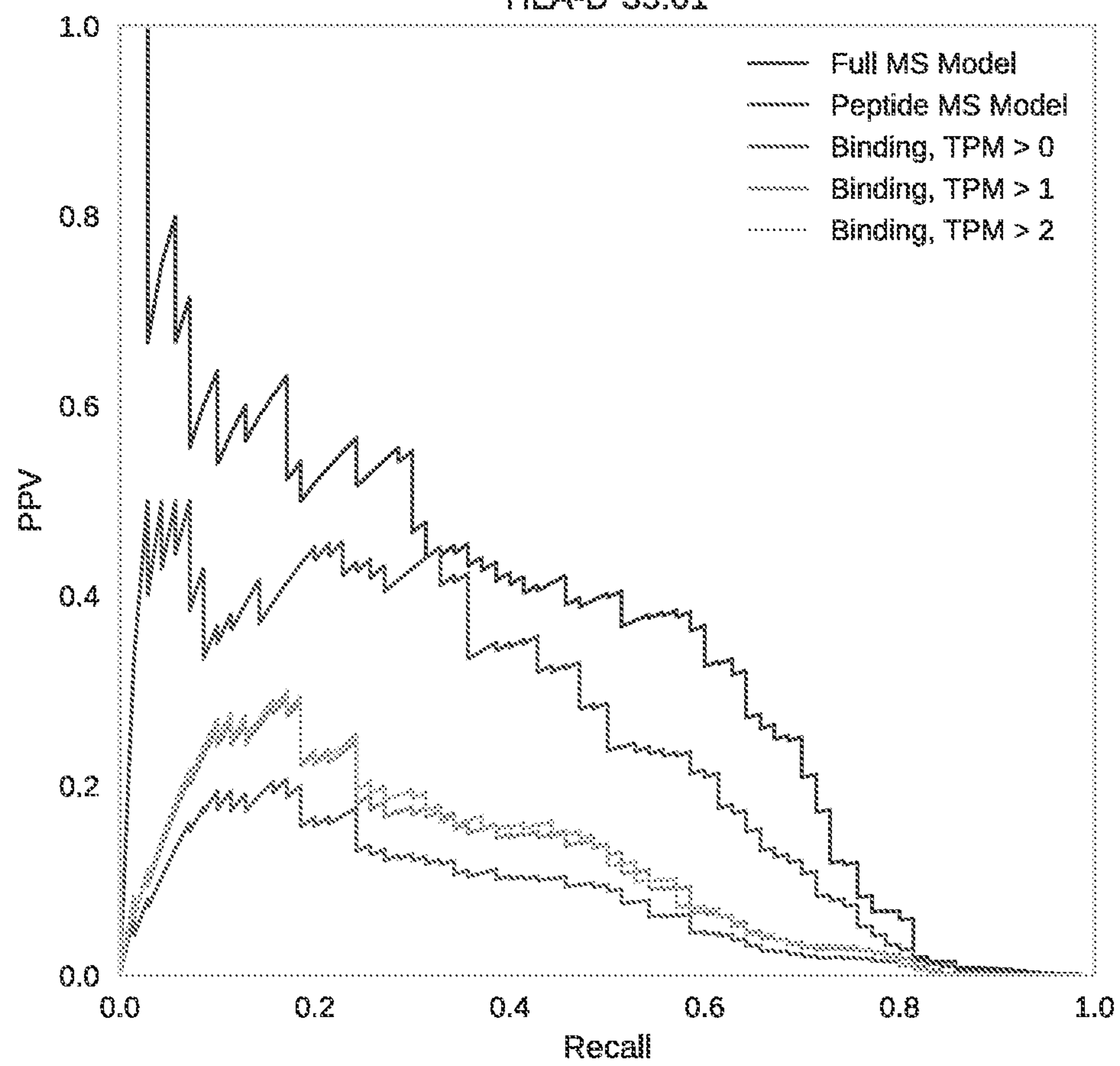
FIG. 17Q HLA-B*35:01
