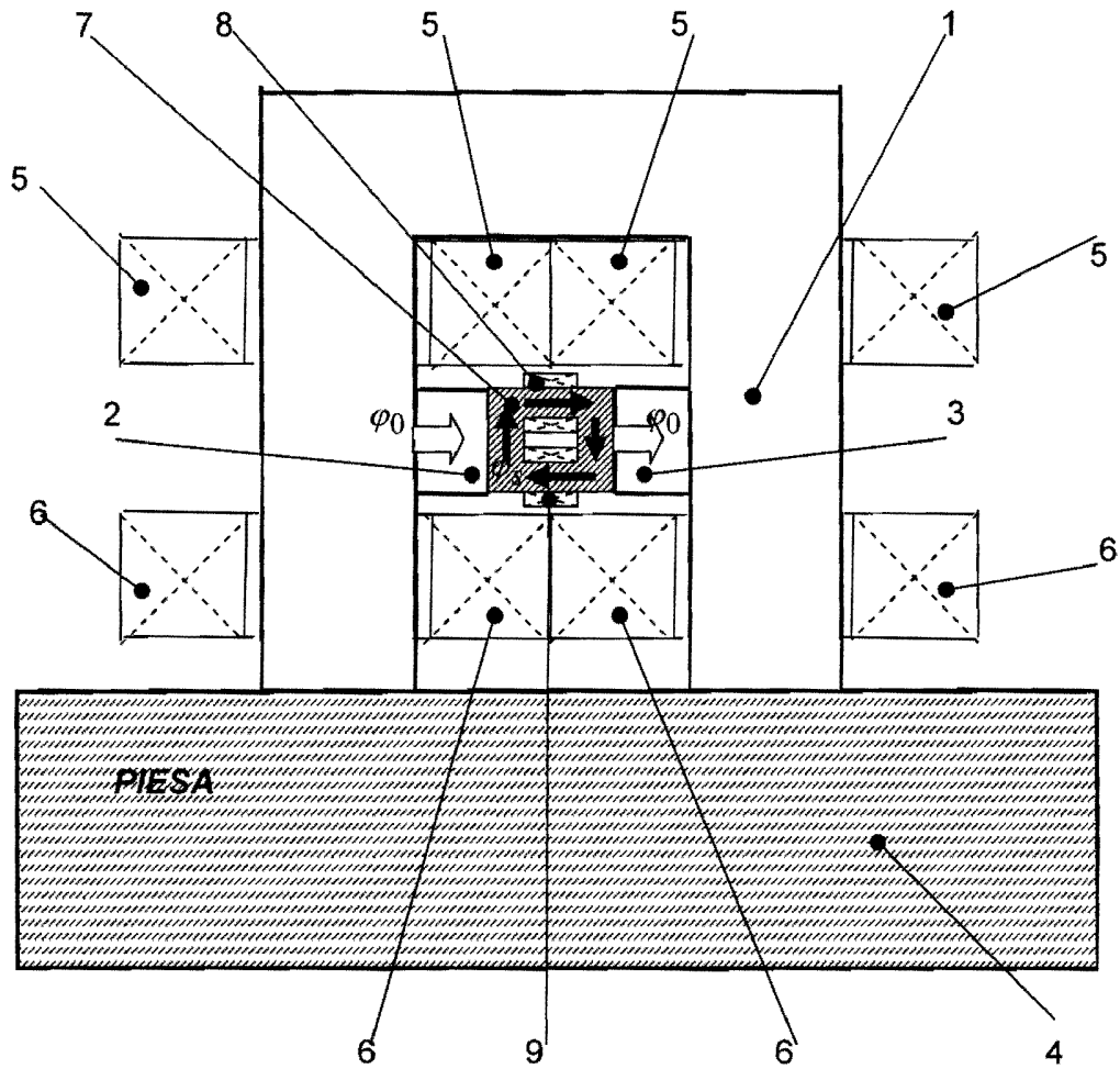
Fig.2, Jug median fara intrefier
