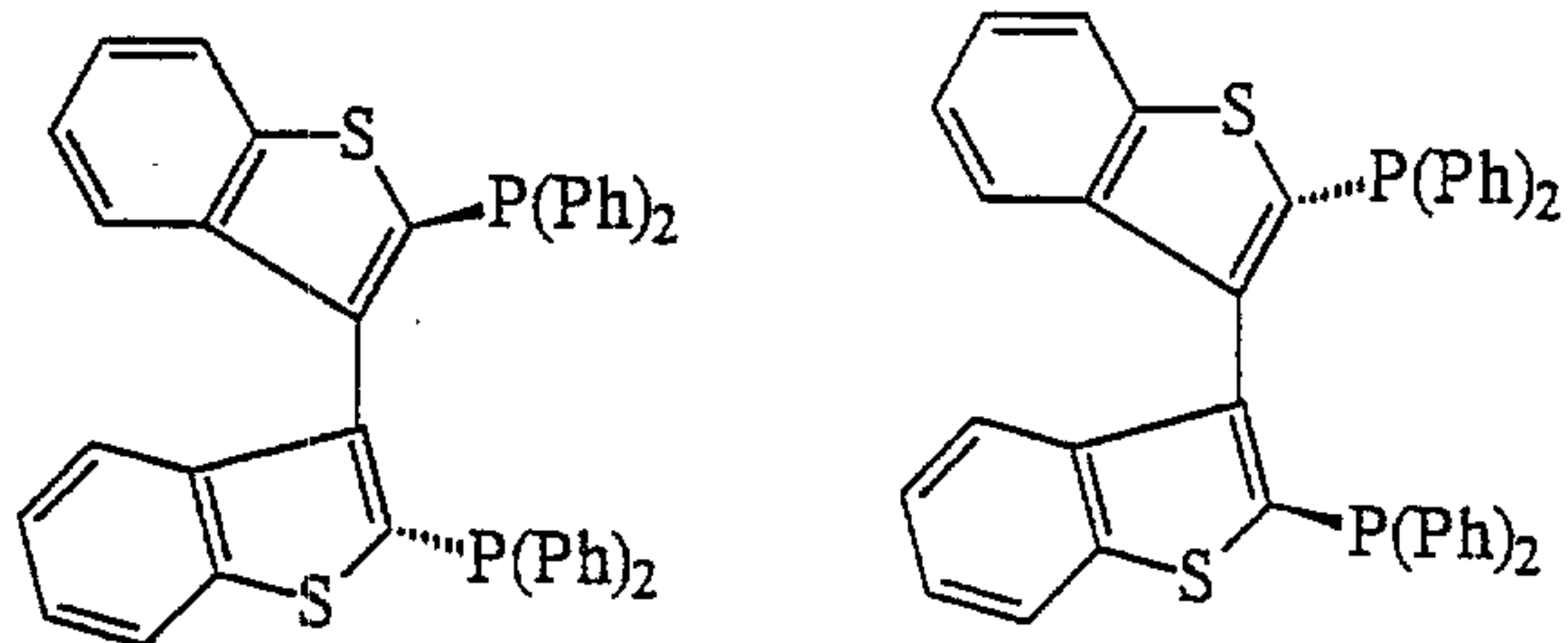
(VII S)
