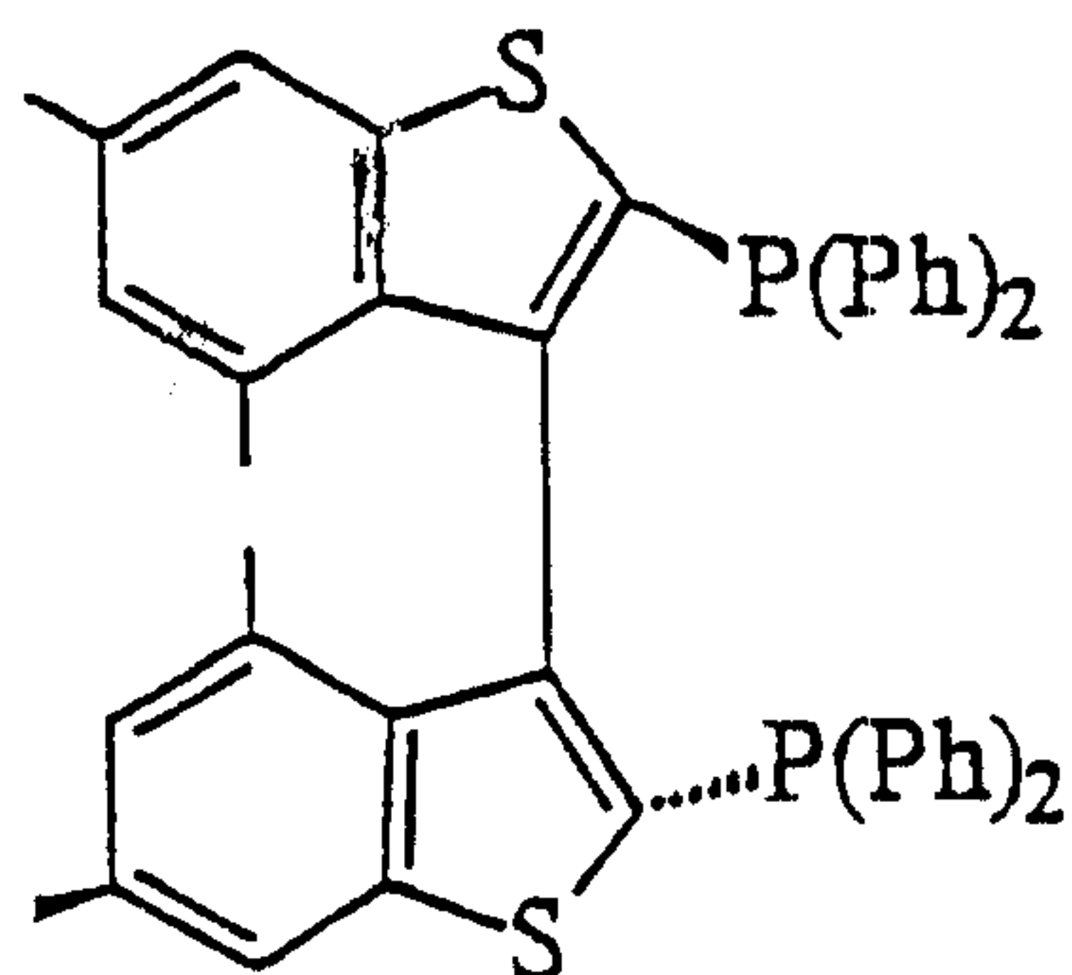
(III R)
