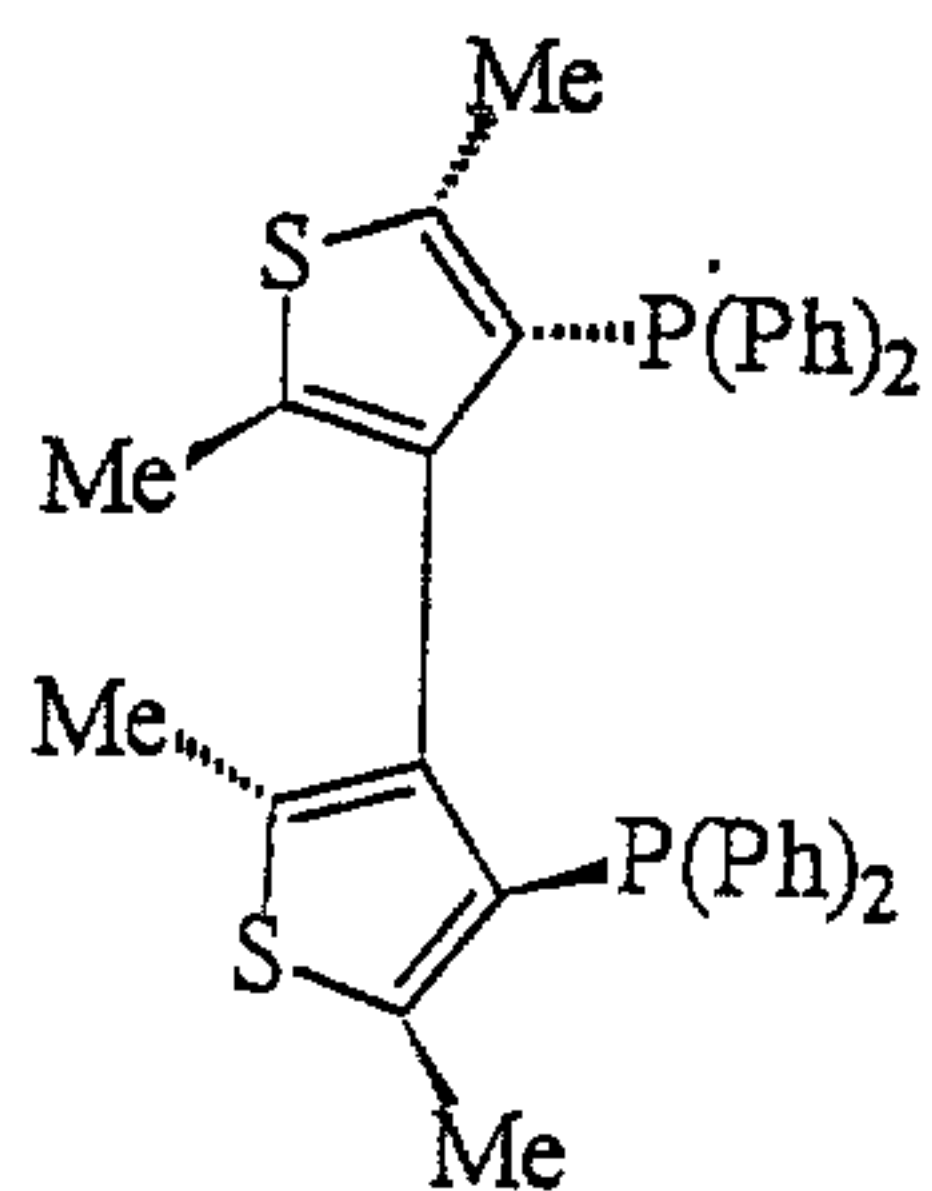
(IV S)
