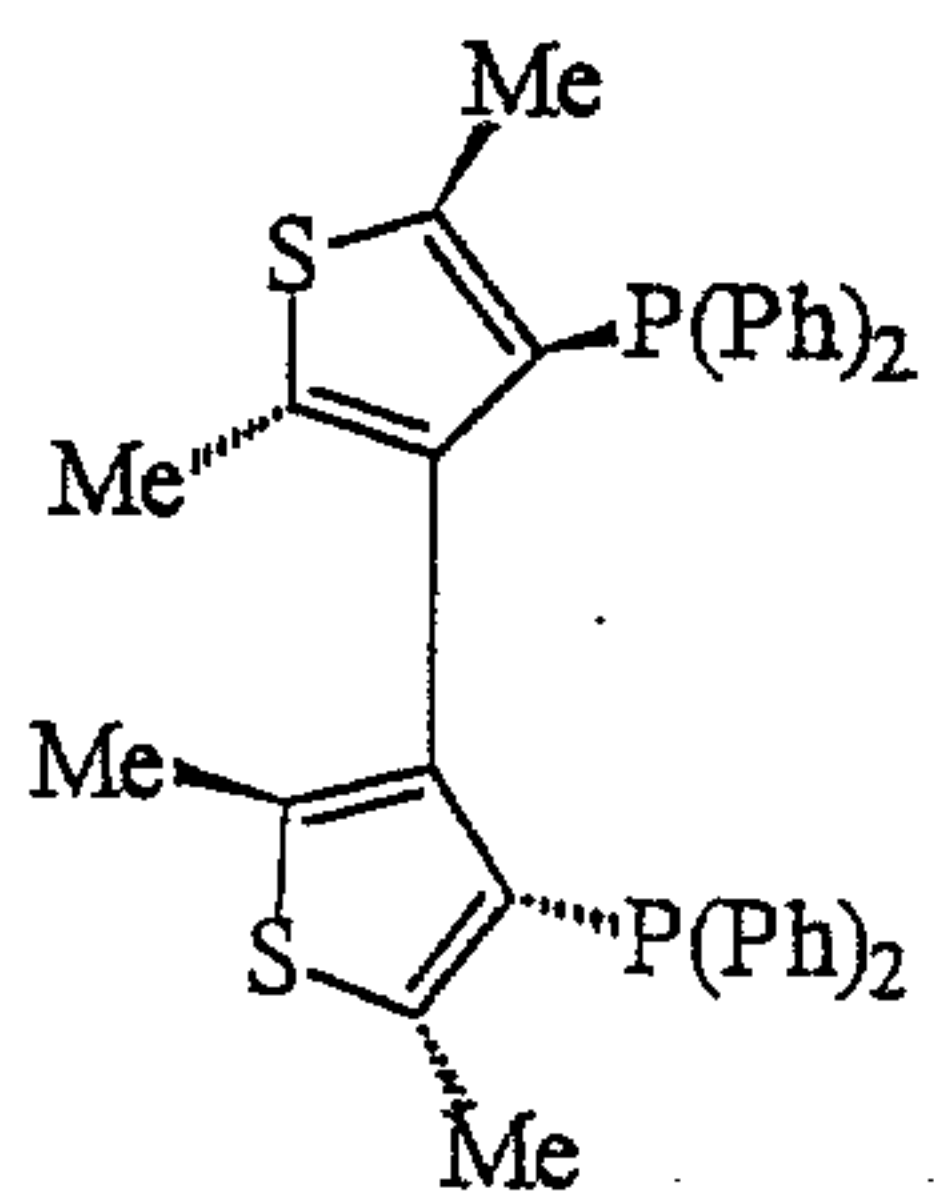
(IV R)
