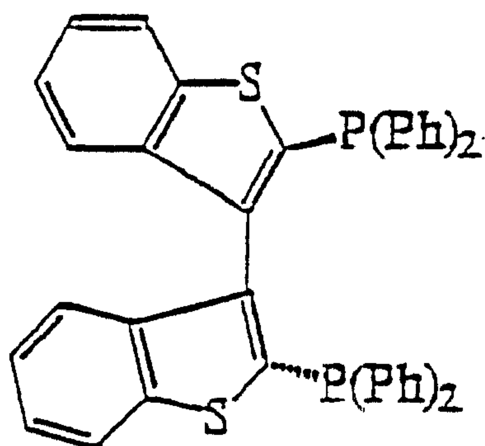
(VIIR)
