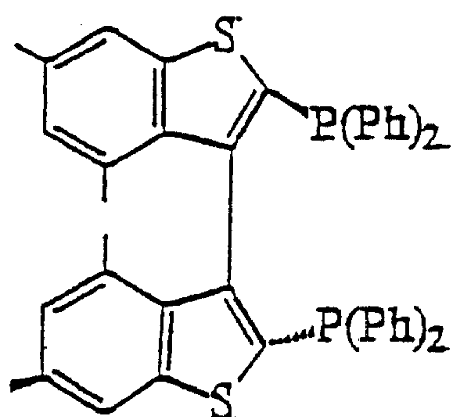
(III R)
