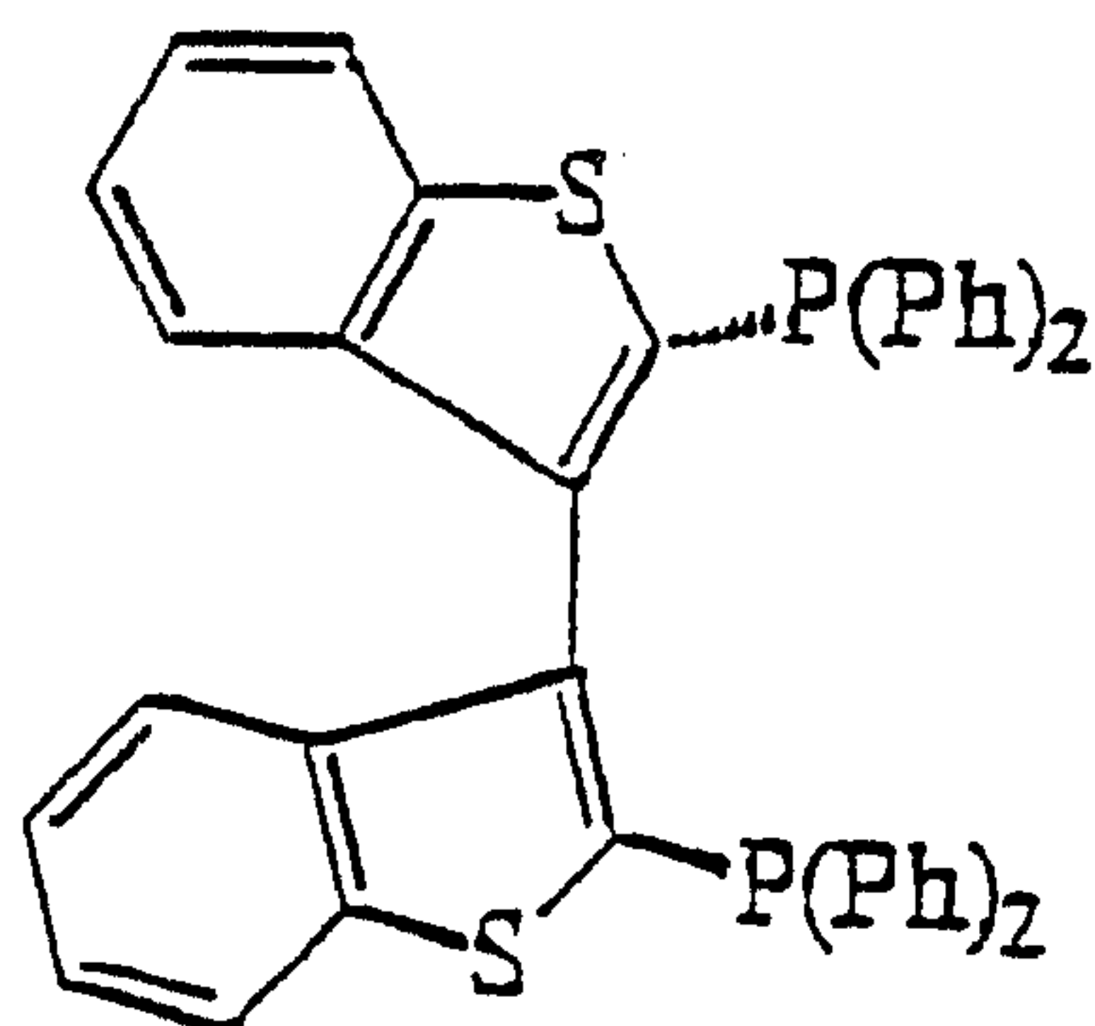
(VIIS)
