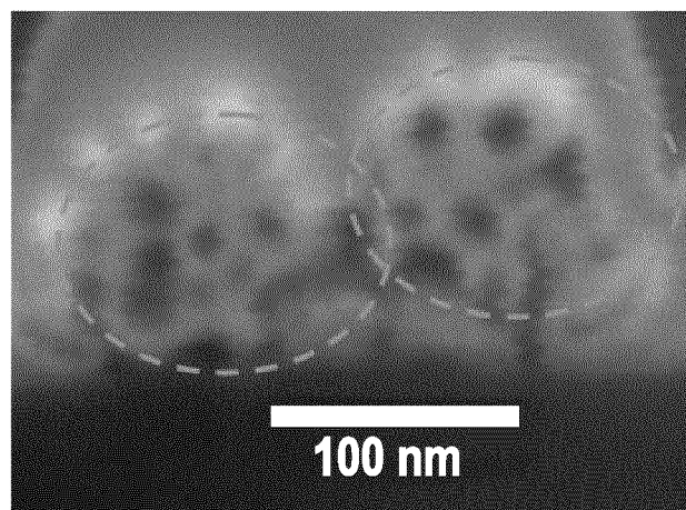
Cross-Sectional SEM
