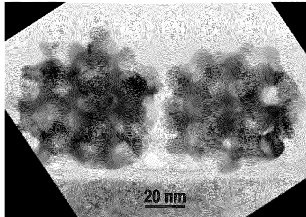
BF-TEM
