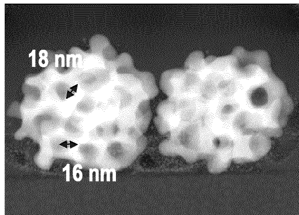
HAADF-STEM
