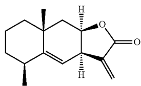
Alantolactone
