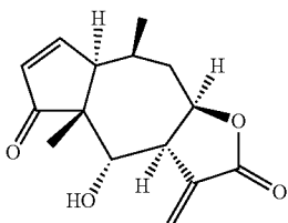
Helenalin
