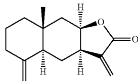
Isoalantolactone
