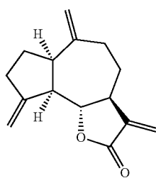
Dehydrocostuslactone
