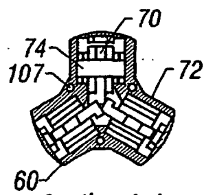
Section A-A FIG. 10B
