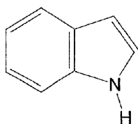
indole
