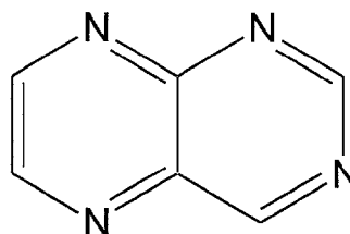
pteridine
