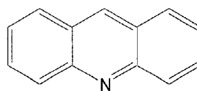
acridine
