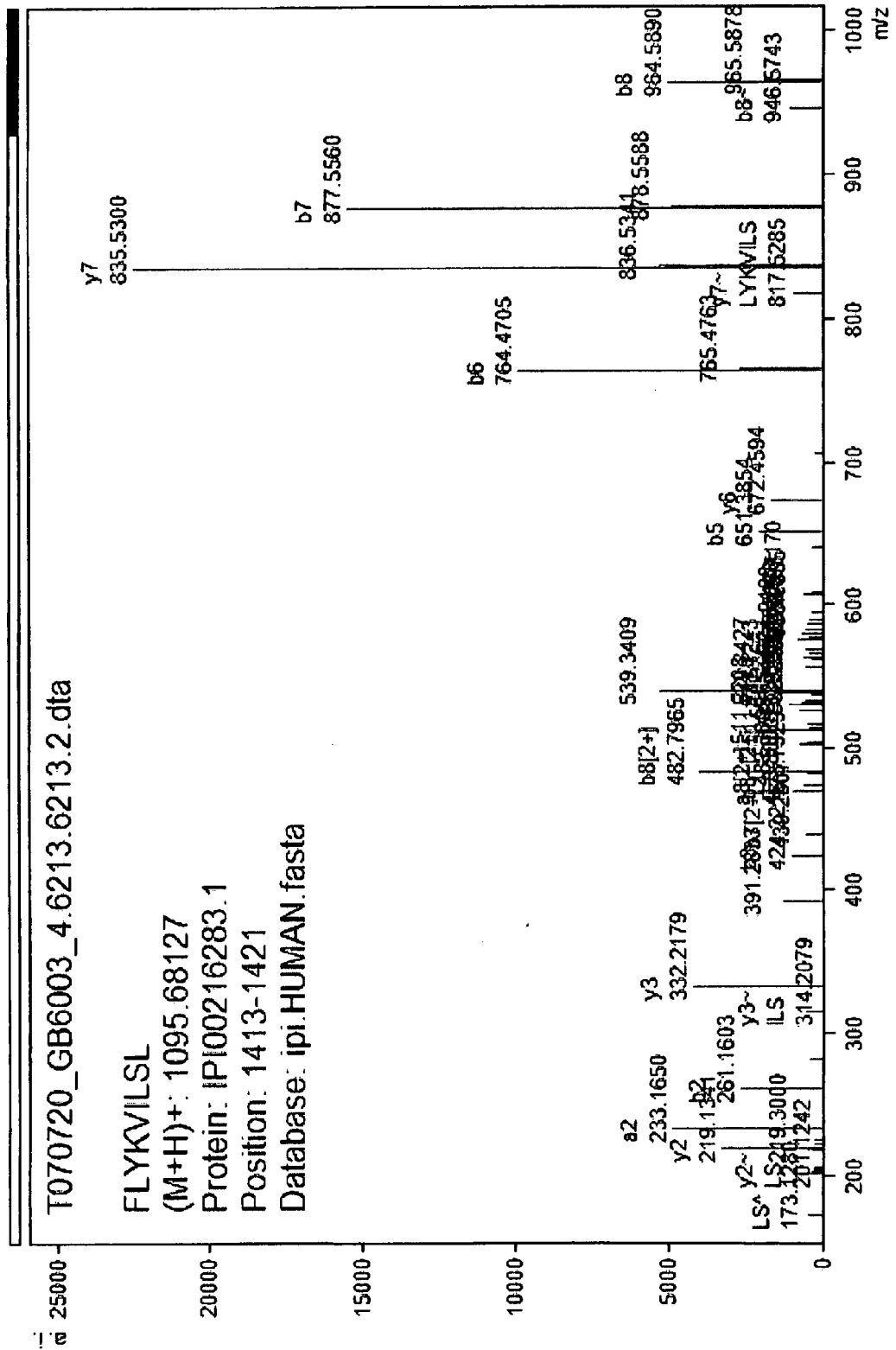
Fig. 1b: PTP-002 (GB6003)
