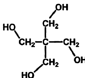
pentaerythritol
