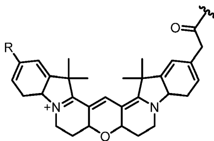
(Dye 106),
