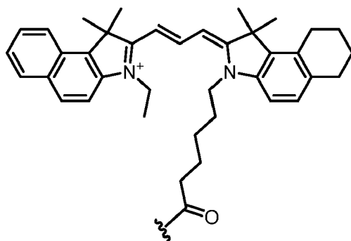
(Dye 105),
