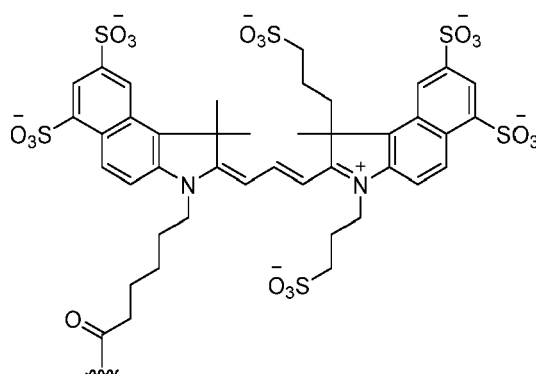
(Dye 101),
