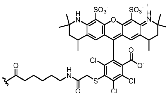
(Dye 103),
