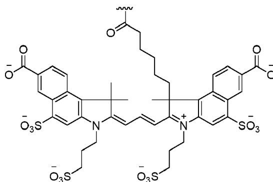
(Dye 102),
