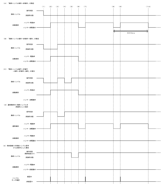
(図467) &lt;遠征時の自動発射に関する作図面&gt;
