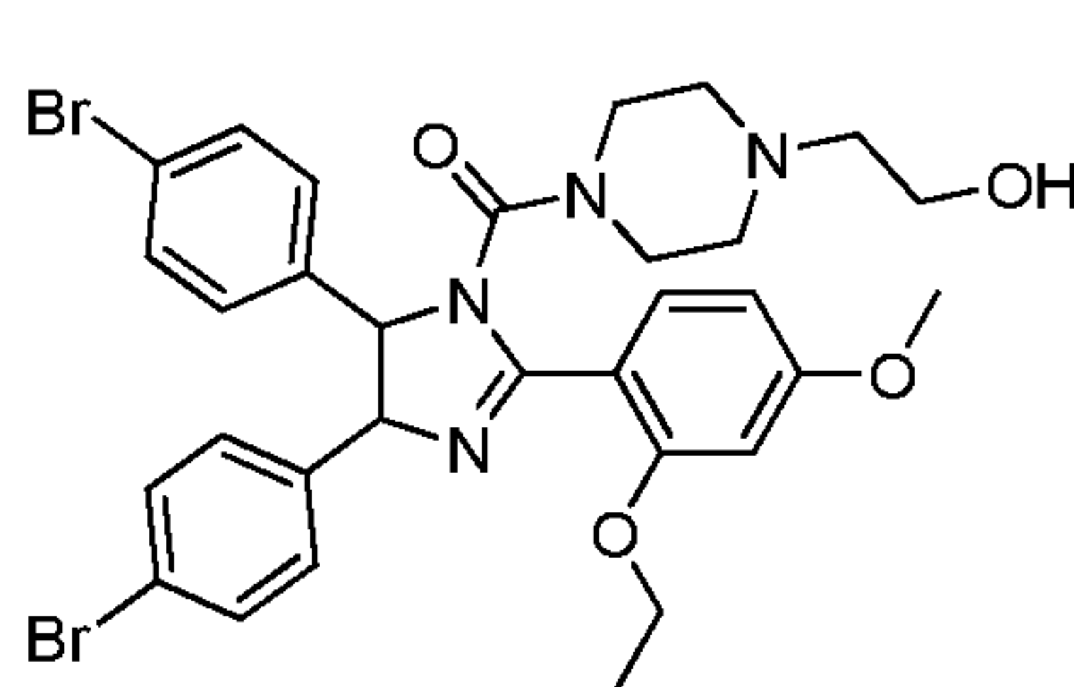
Nutlin-2
