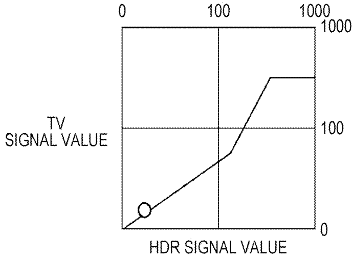
FIG. 27B
