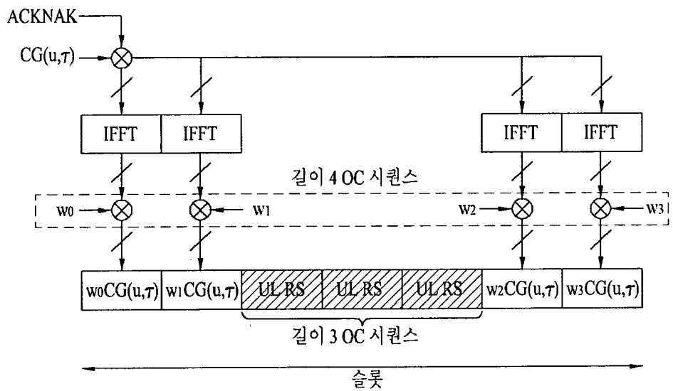
PUCCH 포맷 1a 및 1b 구조 (정상 CP 케이스)
