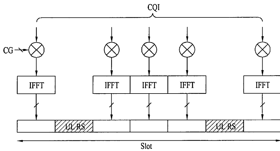
PUCCH 포맷 2, 2a 및 2b 구조 (정상 CP 케이스)
