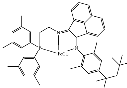
ADiFe XIV
