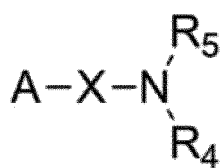
Formule générale (4)
