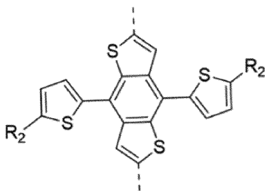
Formule générale (2)
