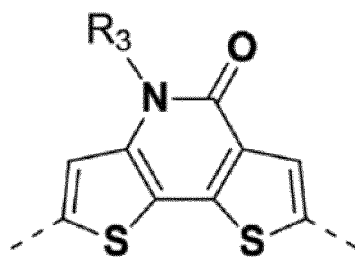
Formule générale (3)
