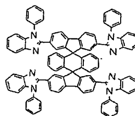
Composé chimique 219
