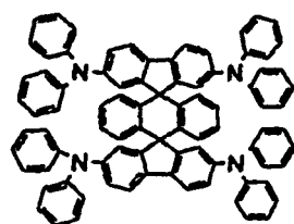
Chemische Verbindung 304
