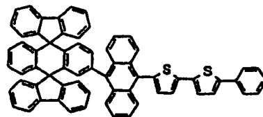
Chemische Verbindung 133
