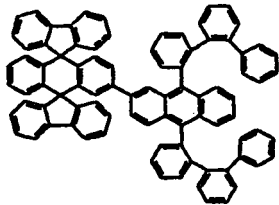
Chemische Verbindung 136
