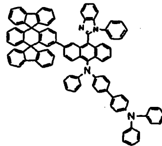
Chemische Verbindung 125
