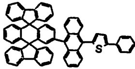
Chemische Verbindung 134
