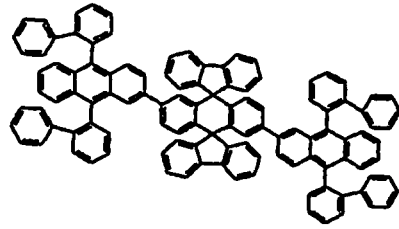
Chemische Verbindung 121
