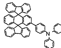
Composé chimique 303
