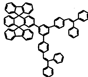
Chemische Verbindung 108
