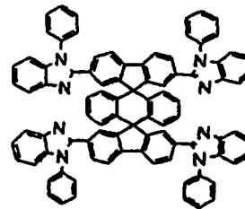
Chemische Verbindung 219
