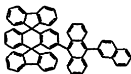
Chemische Verbindung 110
