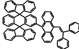
Chemische Verbindung 137
