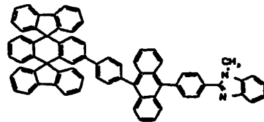
Chemische Verbindung 211
