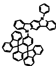
Chemische Verbindung 410
