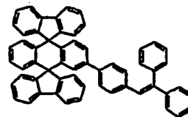
Chemische Verbindung 107
