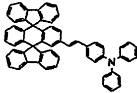
Chemische Verbindung 400
