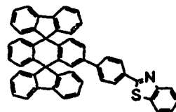
Chemische Verbindung 213
