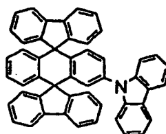
Chemische Verbindung 10
