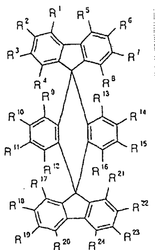
Formule chimique 1
