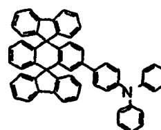
Chemische Verbindung 303
