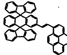
Chemische Verbindung 103
