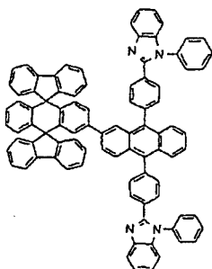
Composé chimique 206
