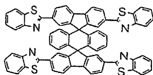
Composé chimique 218
