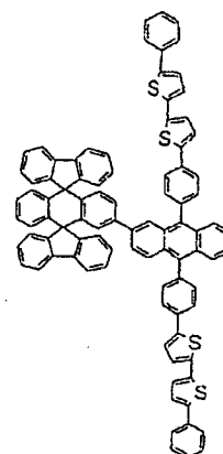
Composé chimique 129
