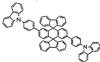
Composé chimique 402
