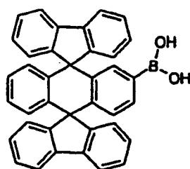
Chemische Verbindung 8
