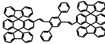
Chemische Verbindung 101
