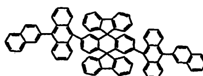
Chemische Verbindung 115
