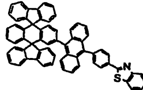
Chemische Verbindung 217
