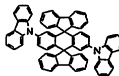
Chemische Verbindung 407
