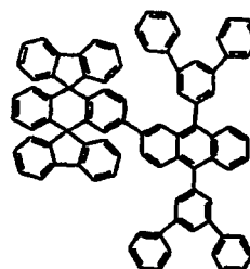
Chemische Verbindung 119
