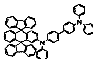
Chemische Verbindung 307
