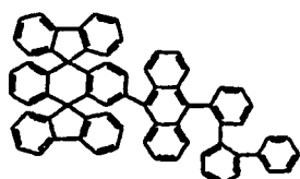
Chemische Verbindung 112
