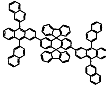
Chemische Verbindung 123
