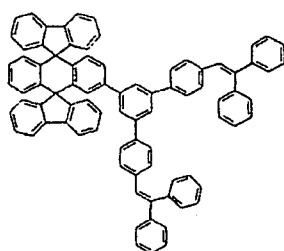
Composé chimique 108
