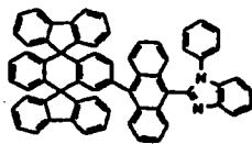
Chemische Verbindung 200
