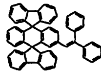
Chemische Verbindung 106
