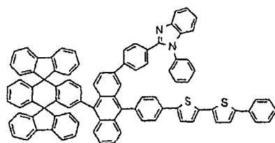
Composé chimique 132
