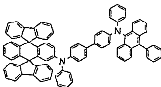
Composé chimique 408
