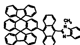
Chemische Verbindung 205
