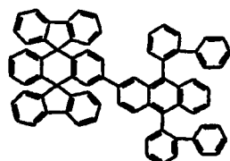
Chemische Verbindung 118
