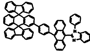
Chemische Verbindung 207
