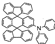
Composé chimique 11
