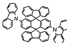
Composé chimique 407
