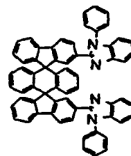
Chemische Verbindung 221
