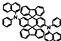
Chemische Verbindung 302
