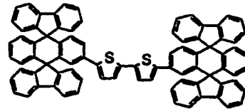
Chemische Verbindung 135
