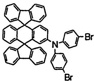
Chemische Verbindung 7
