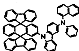
Chemische Verbindung 306
