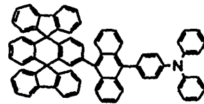
Chemische Verbindung 401
