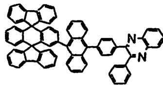
Chemische Verbindung 209
