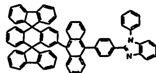
Chemische Verbindung 204
