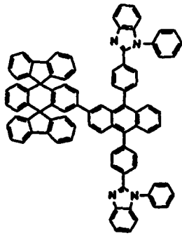
Chemische Verbindung 206
