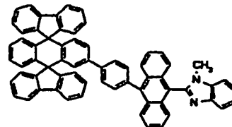
Chemische Verbindung 201
