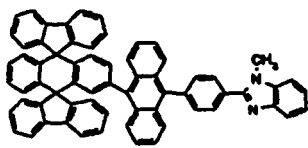
Chemische Verbindung 208
