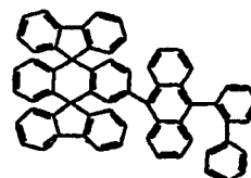
Chemische Verbindung 111
