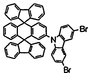
Chemische Verbindung 6
