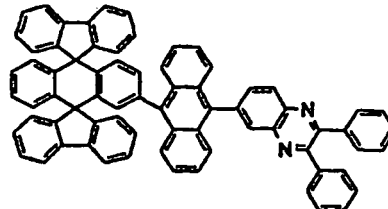
Chemische Verbindung 203
