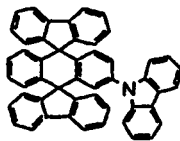
Chemische Verbindung 404
