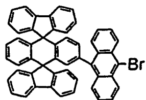
Chemische Verbindung 5
