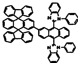
Chemische Verbindung 202
