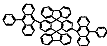
Chemische Verbindung 114
