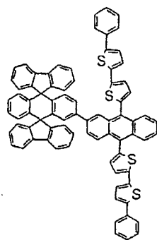
Composé chimique 128
