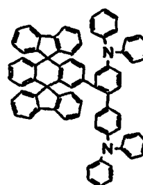
Chemische Verbindung 305
