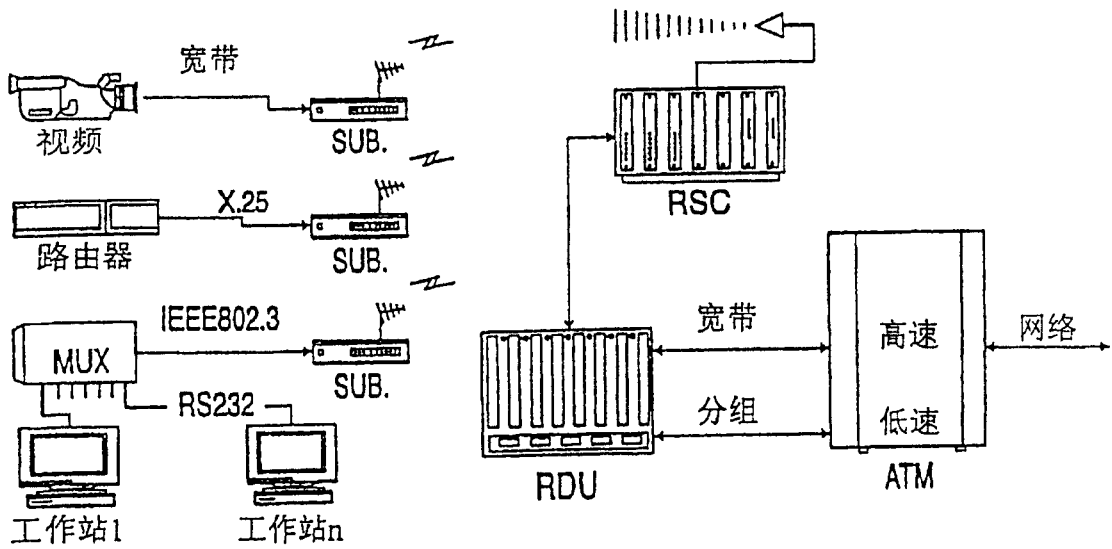
宽带和分组网络接口 图2G
