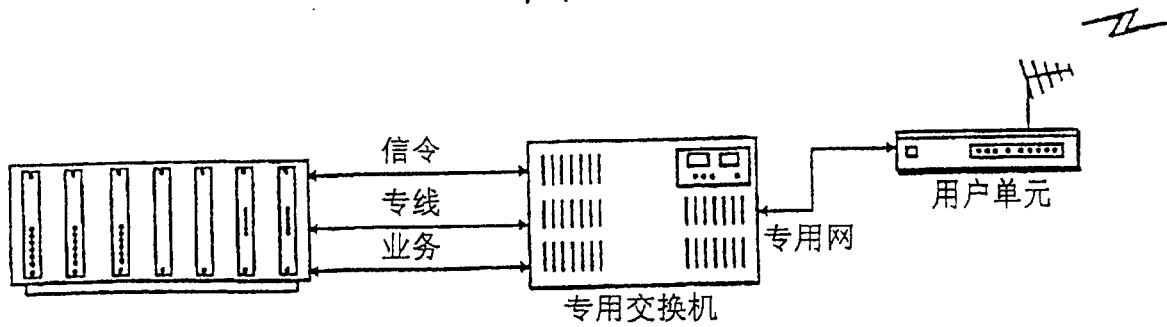
宽带和分组网络接口 图2G
