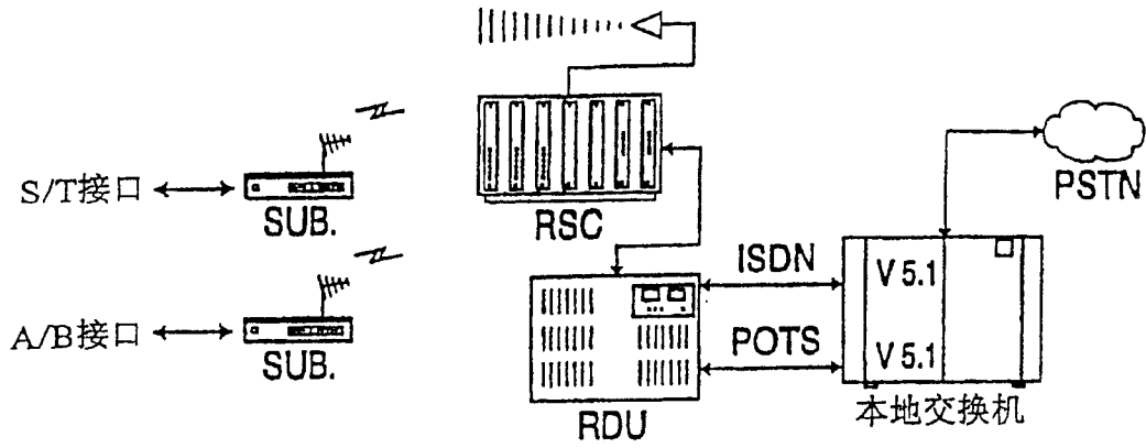
ISDN和POTS网络接口 图2F
