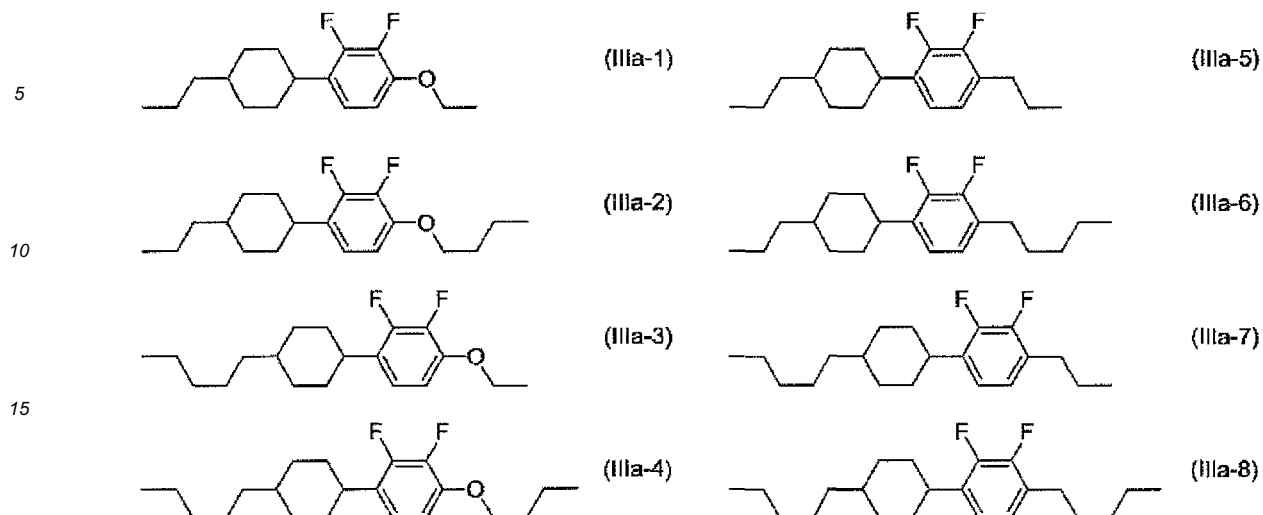
[Chem. 6]
