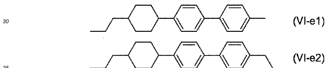
[Chem. 23]
