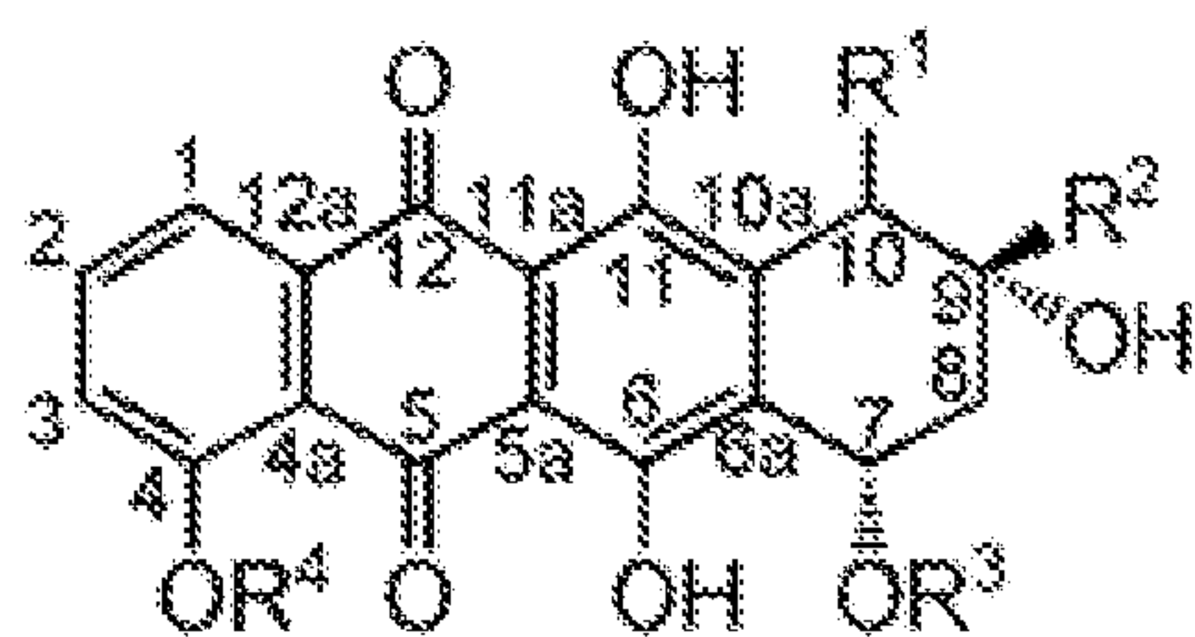
Aglycone
