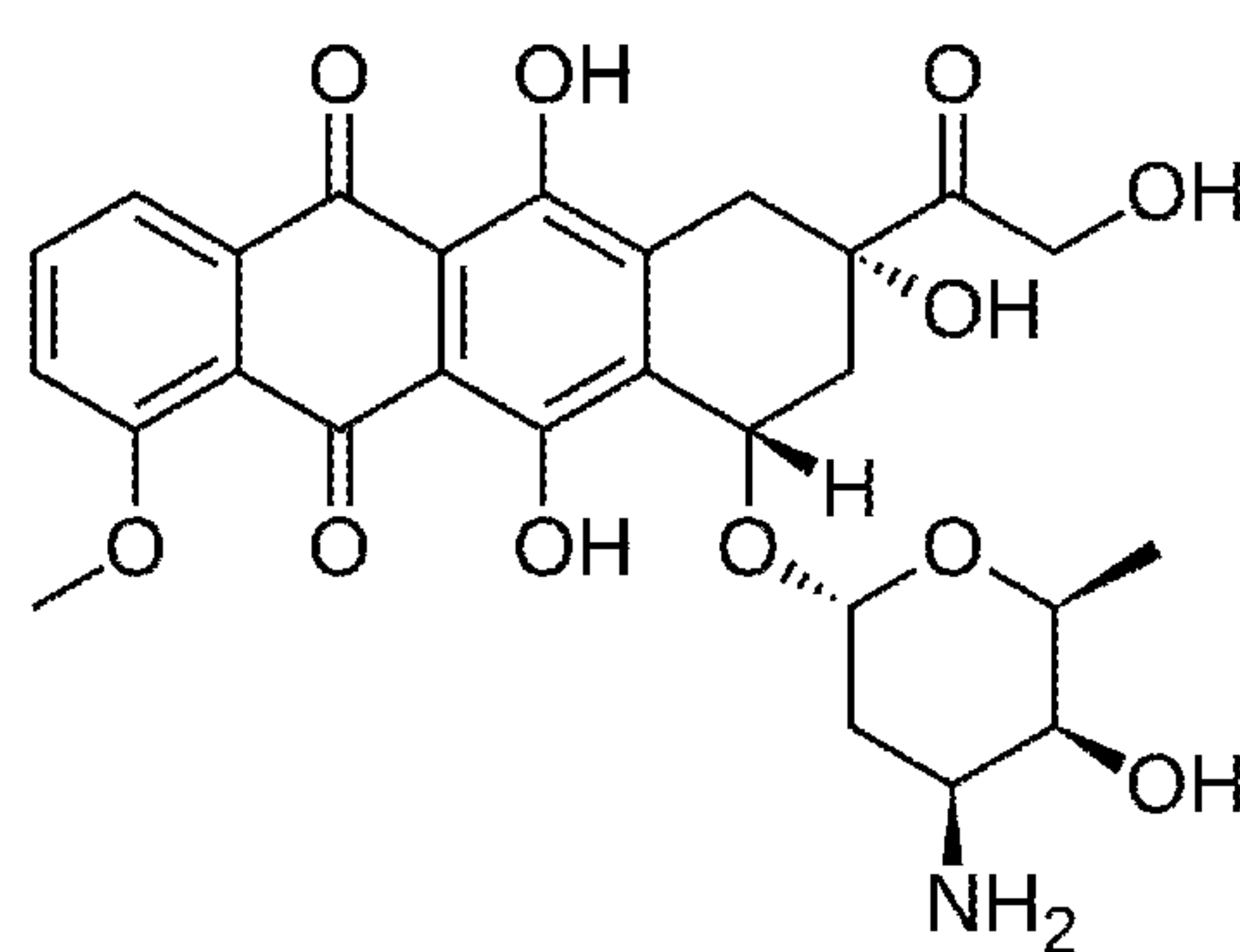
Doxorubicin
