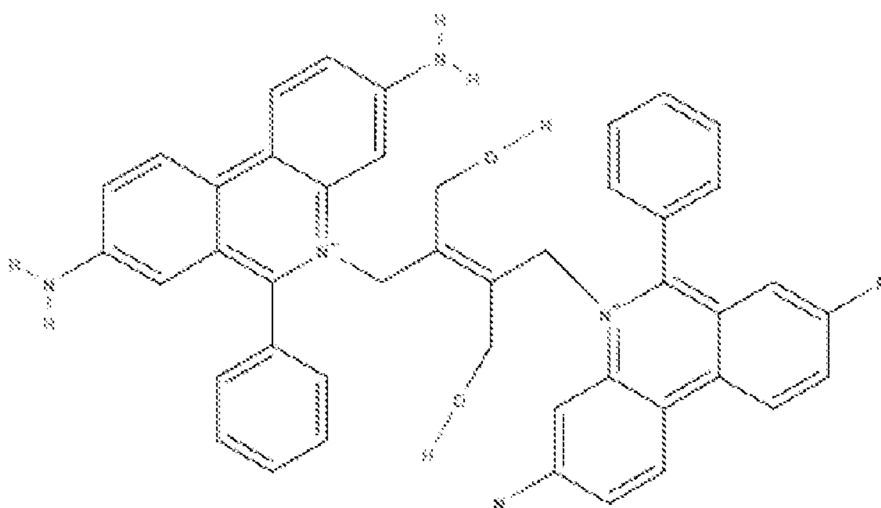
XXIX
