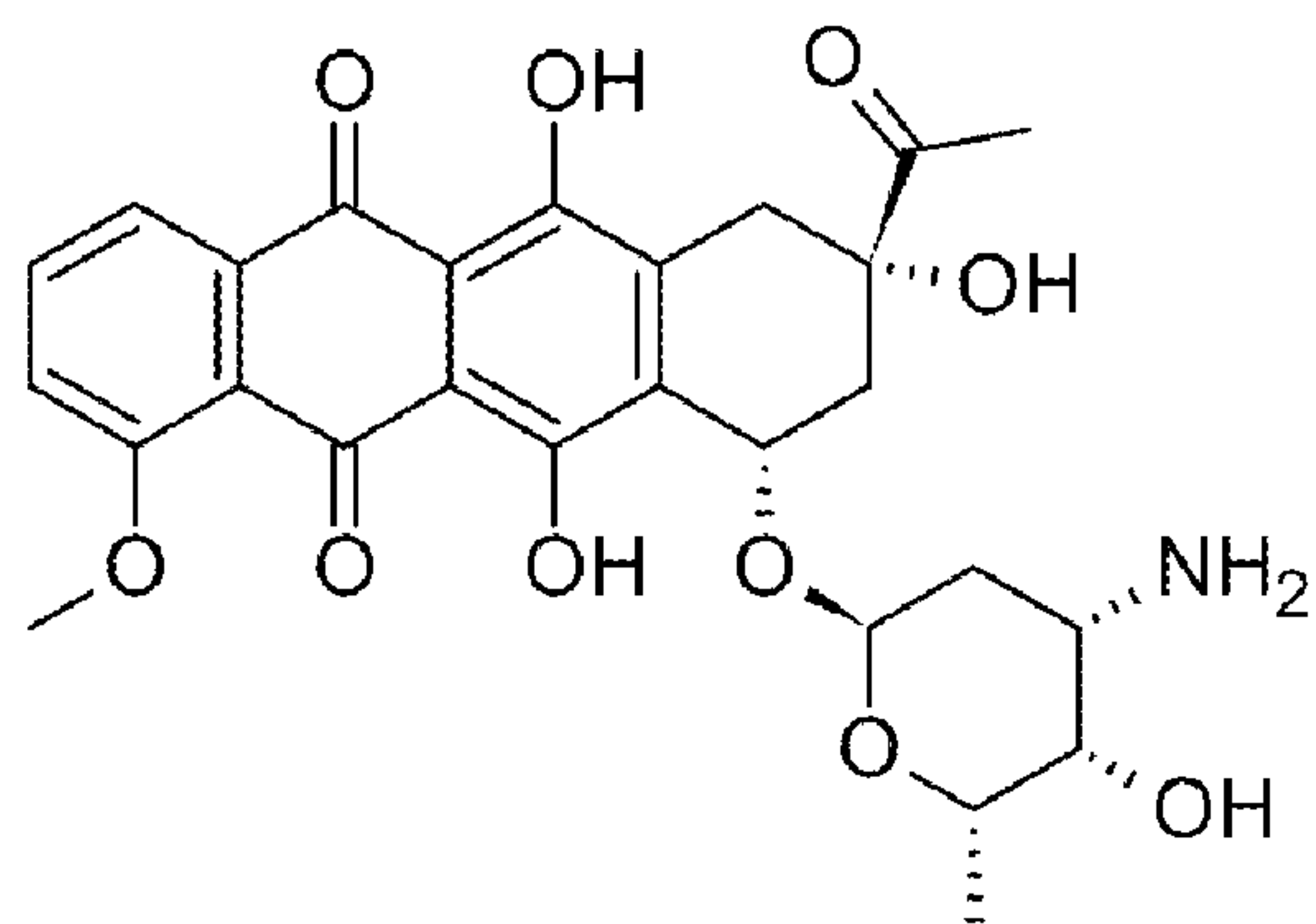
Daunorubicin
