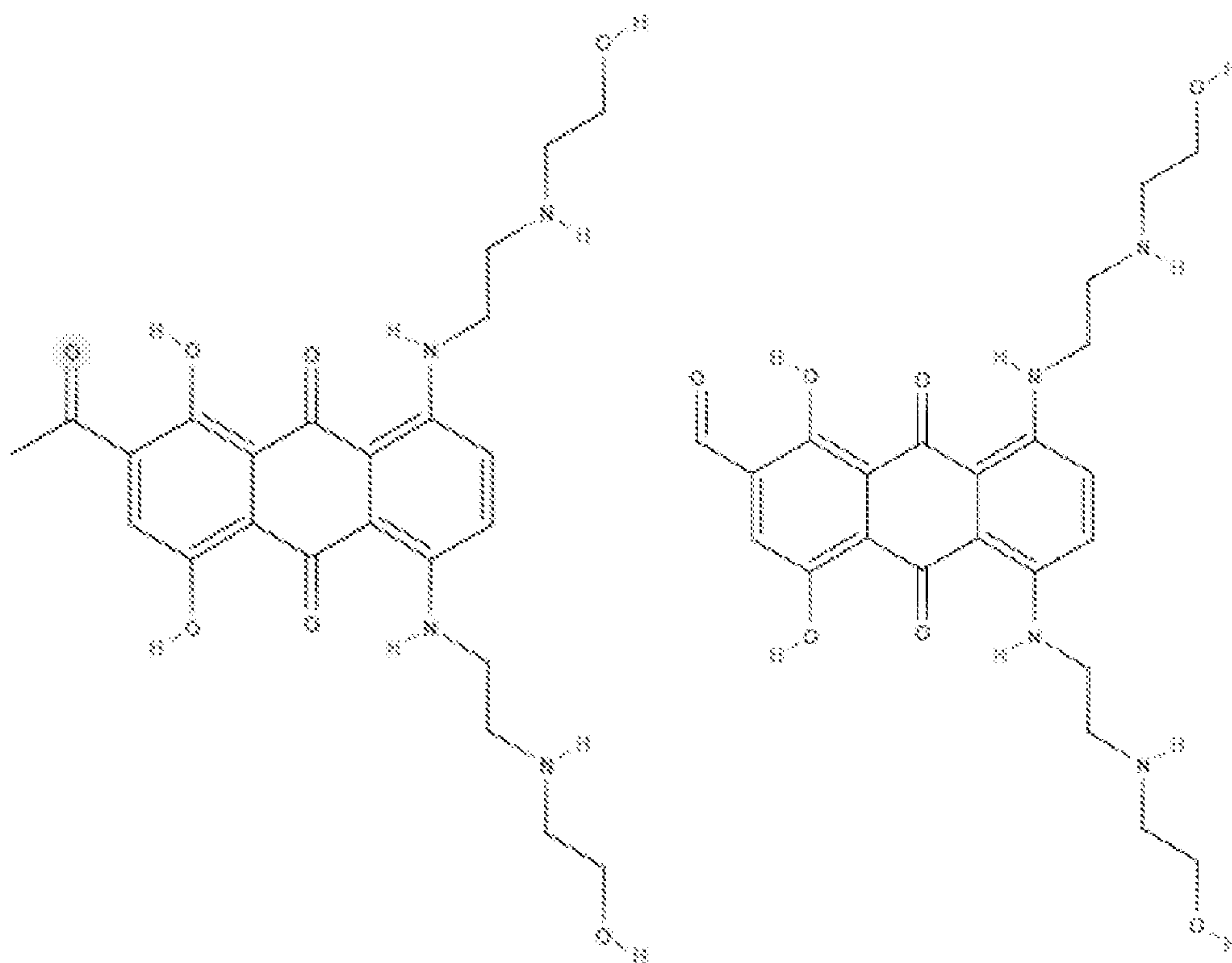
XXXI
