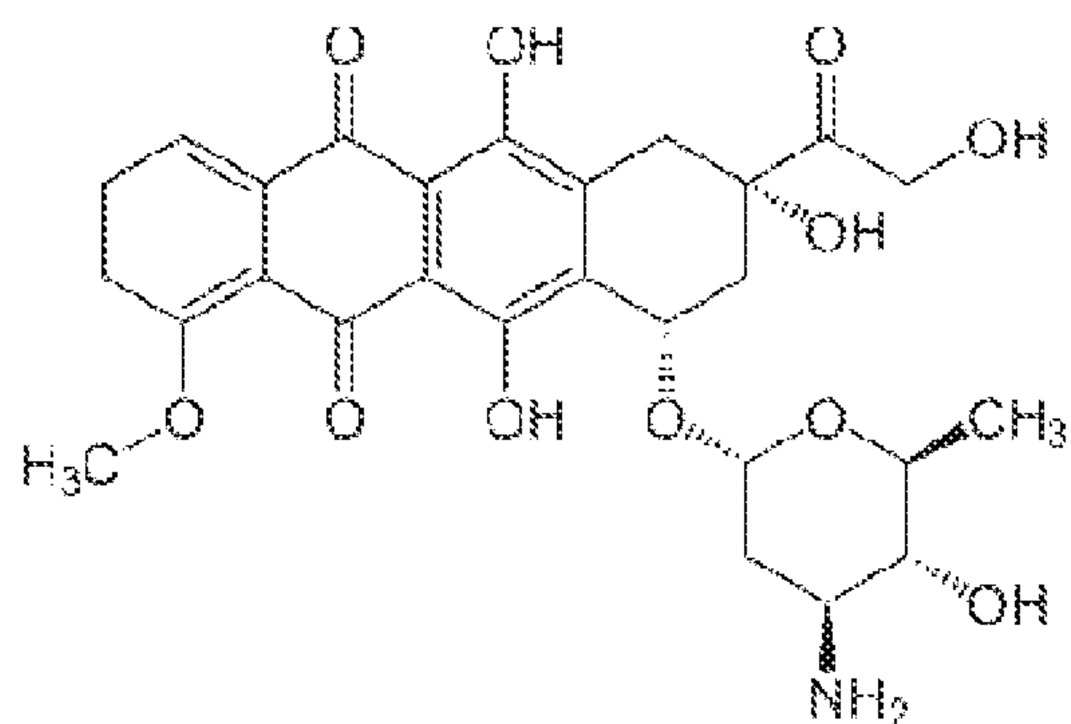
Epirubicin
