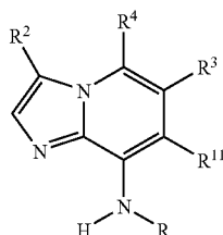
Imidazopyridine
