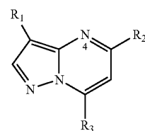
Pyrazolo[1,5-a]pyrimidines
