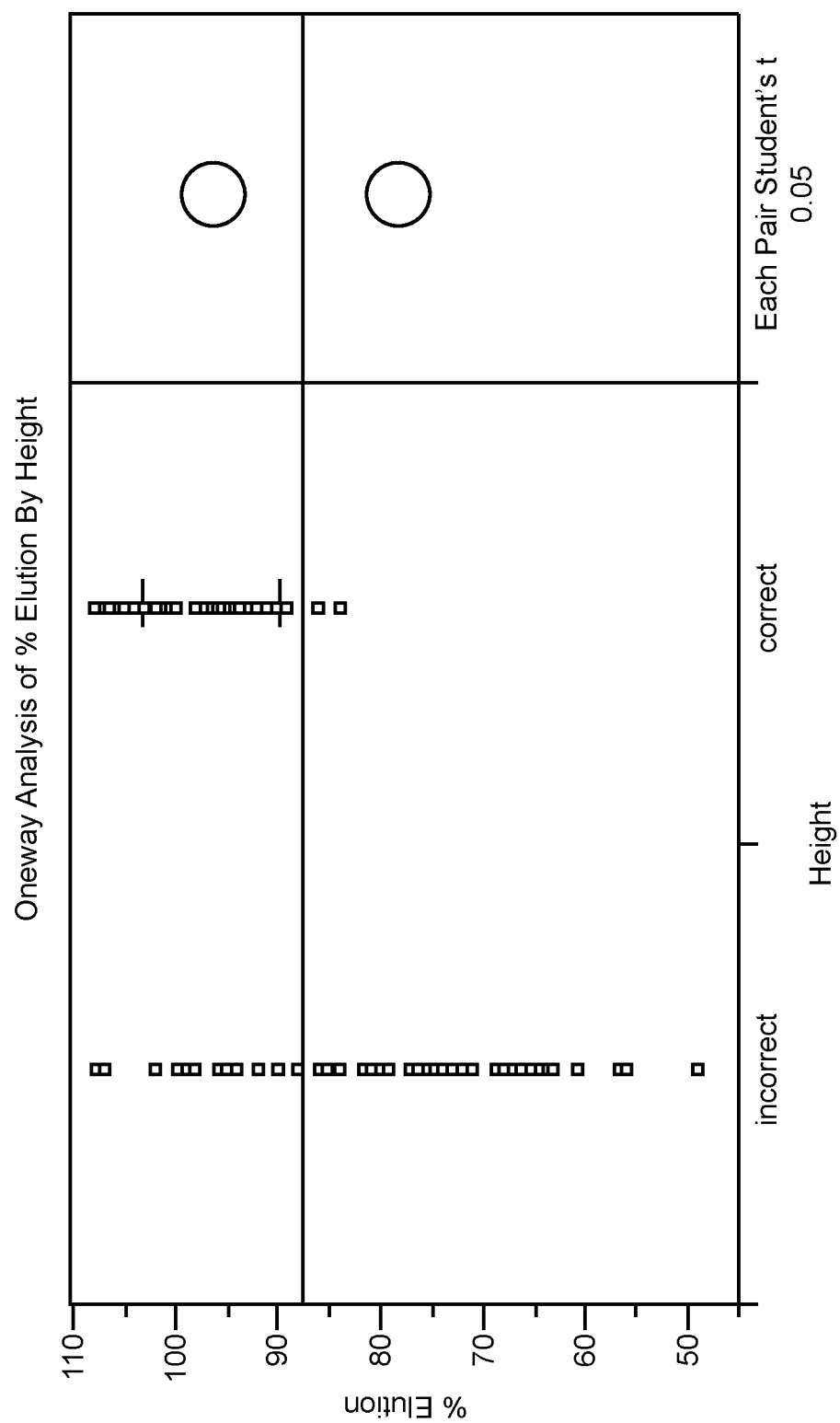
\frac{\infty}{F|G}
