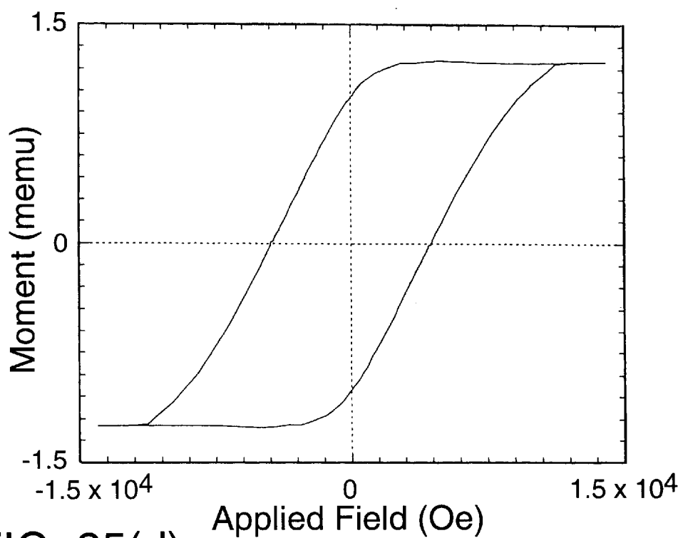
FIG. 25(d) Easy Axis Loop
