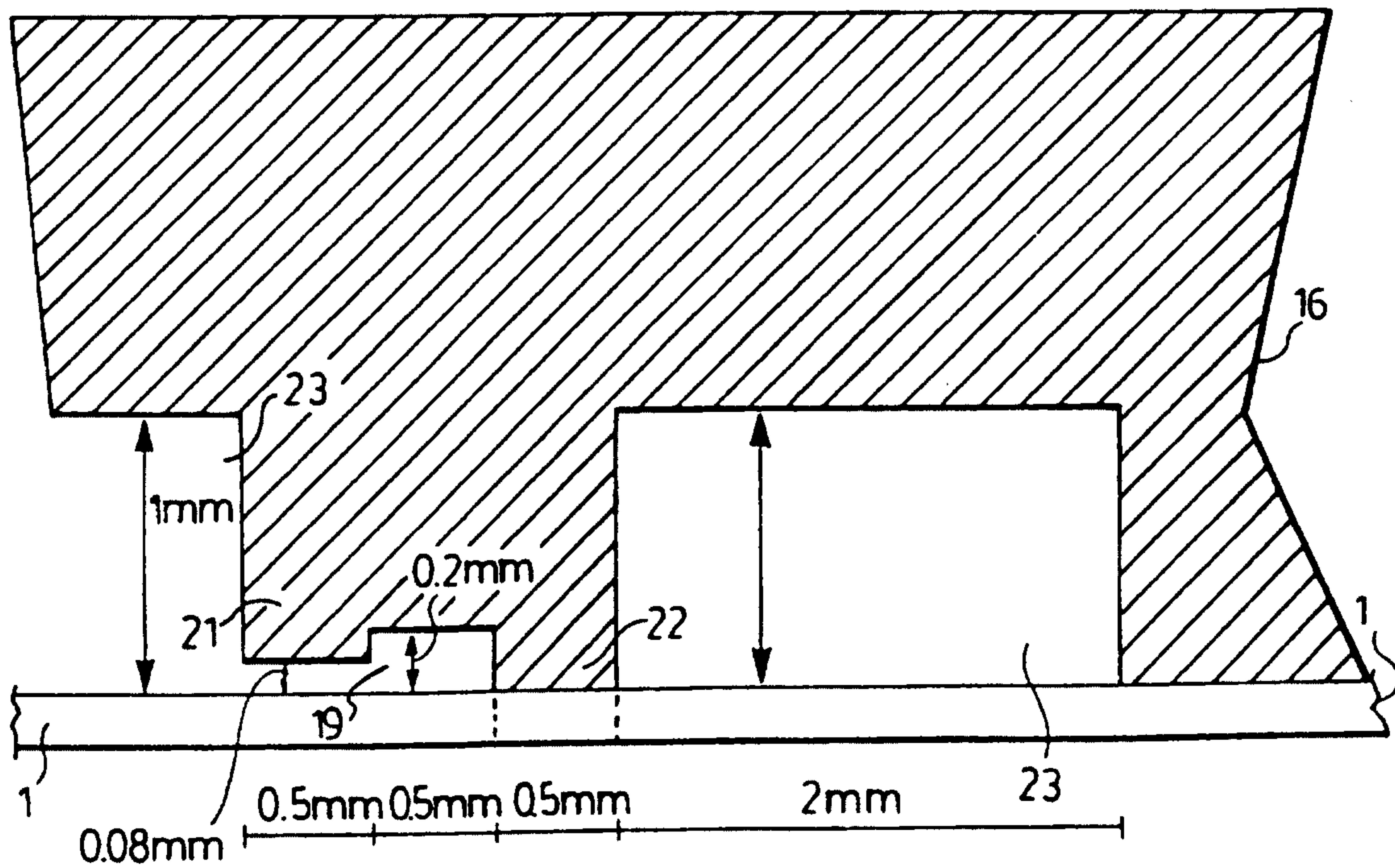
FIG. 23 D-D
