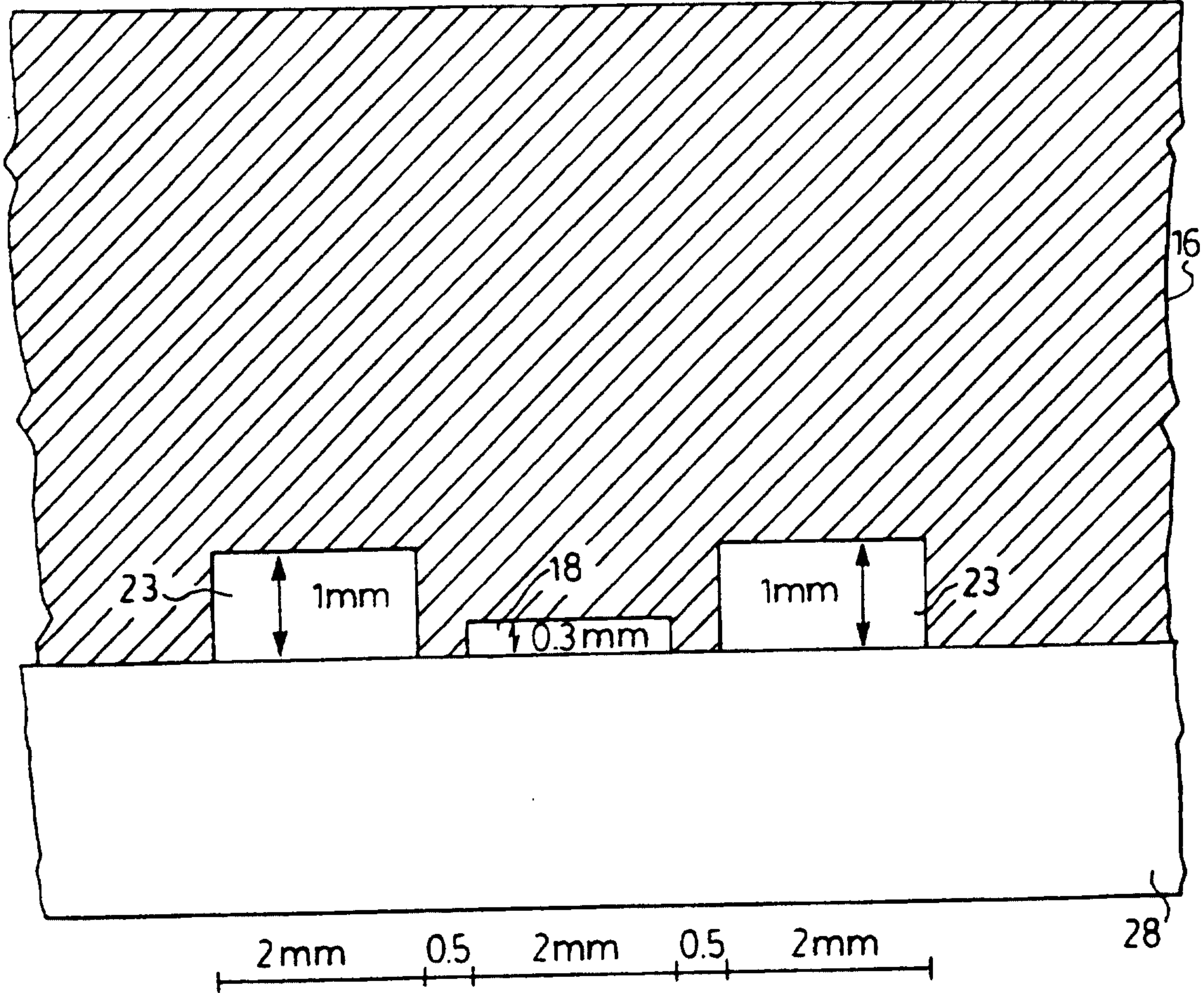
FIG. 21 B-B
