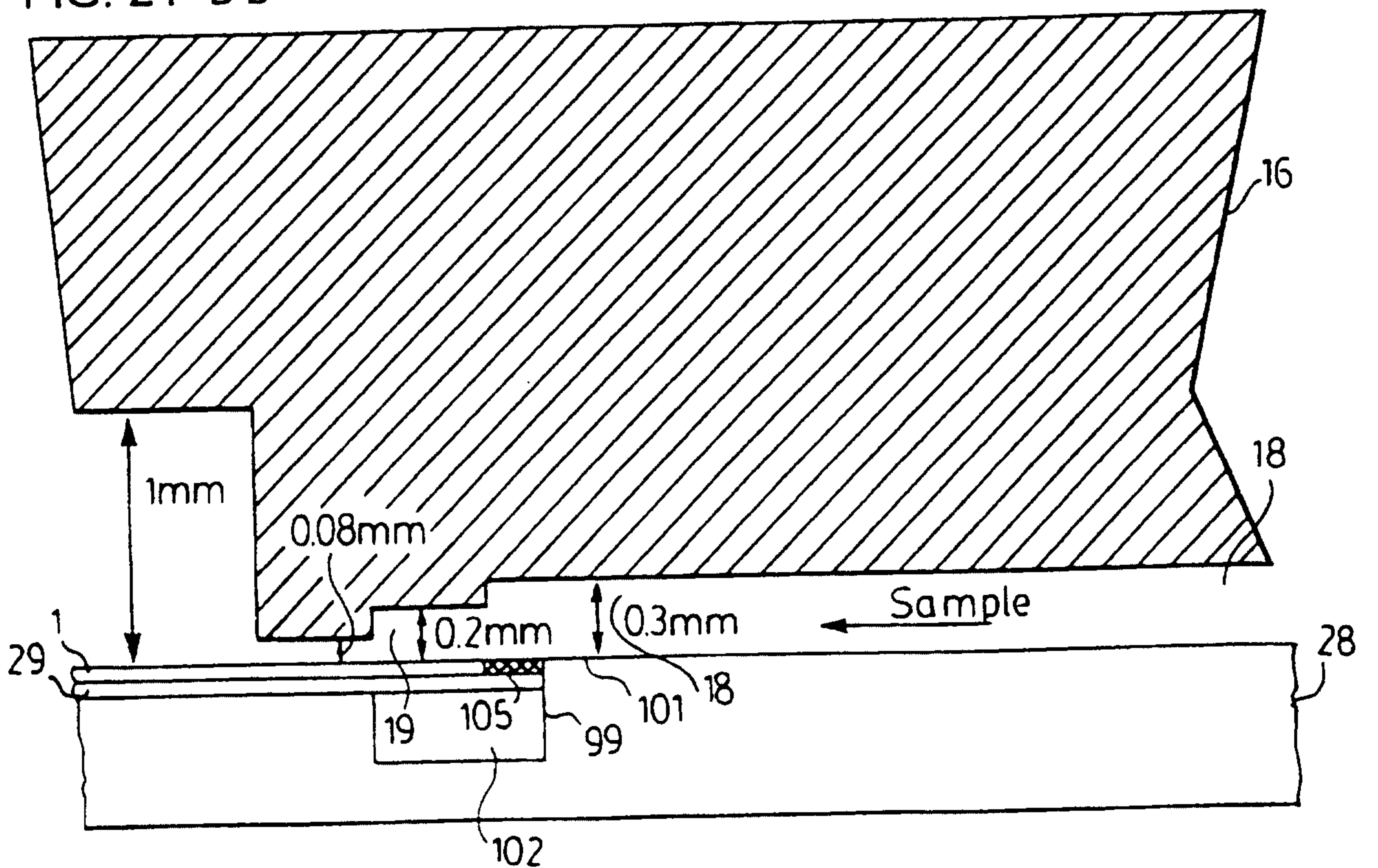
FIG. 21 B-B
