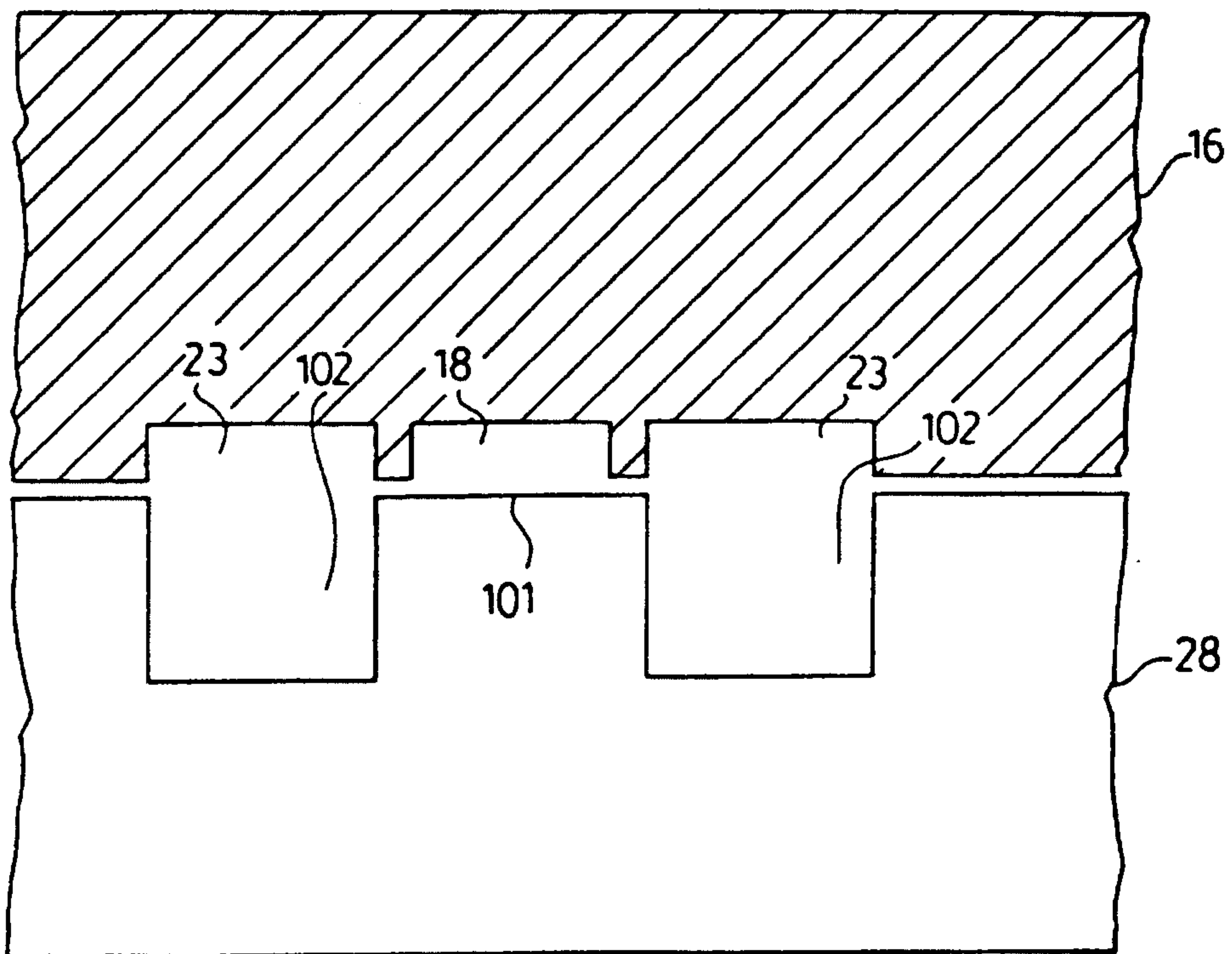
FIG. 22 c-c
