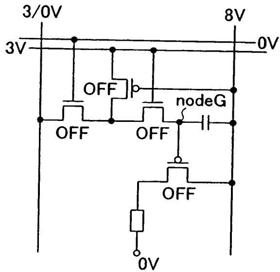
FIG. 9B blank period
