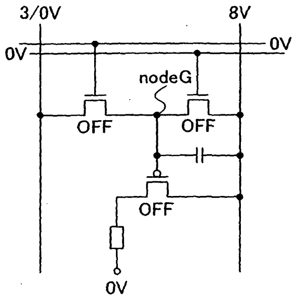
FIG. 3B blank period
