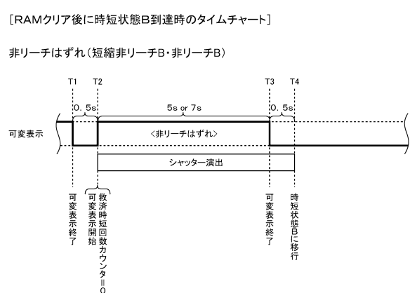
【図 11-22】 [RAMクリア後に時短状態B到達時のタイムチャート]
