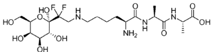
Verbindung 1,
