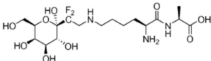
Verbindung 3,
