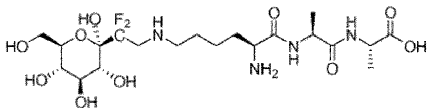
Verbindung 2,
