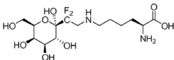
Verbindung 4,
