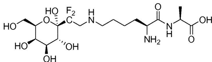
Composé 3,
