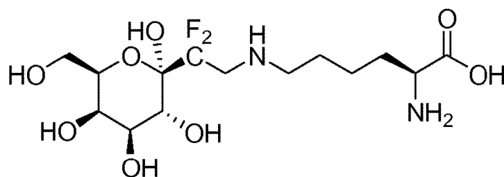
Composé 4,
