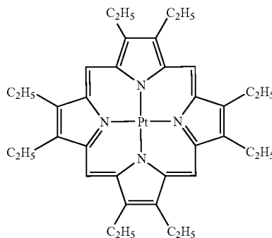
\text{PtOEP}
