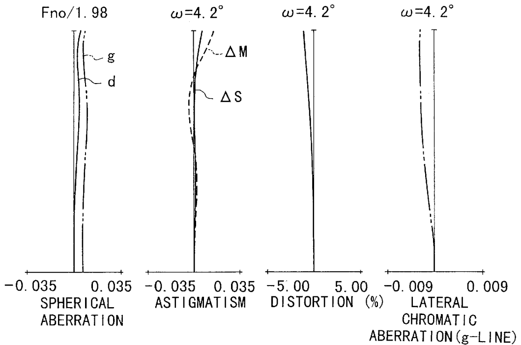
FIG. 24A FIG. 24B FIG. 24C FIG. 24D
