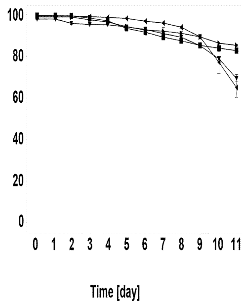
(D) Product Conc. [mg/L]
