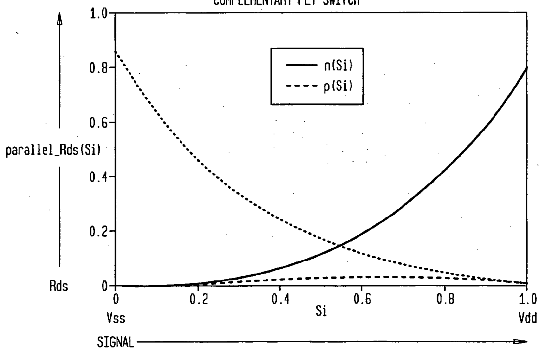
FIG. 241 COMPLEMENTARY FET SWITCH
