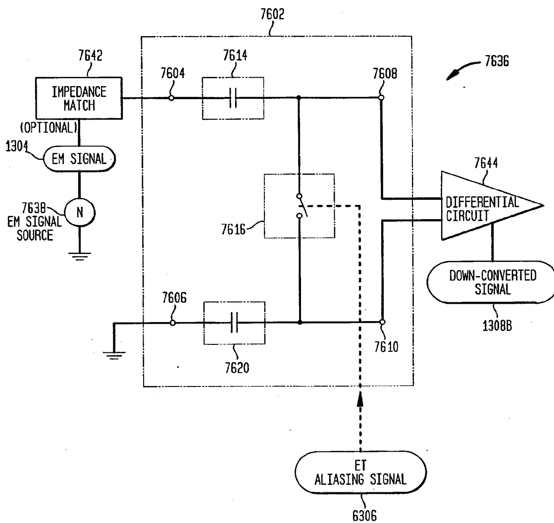
FIG. 76E EXAMPLE INPUT/OUTPUT CIRCUITRY
