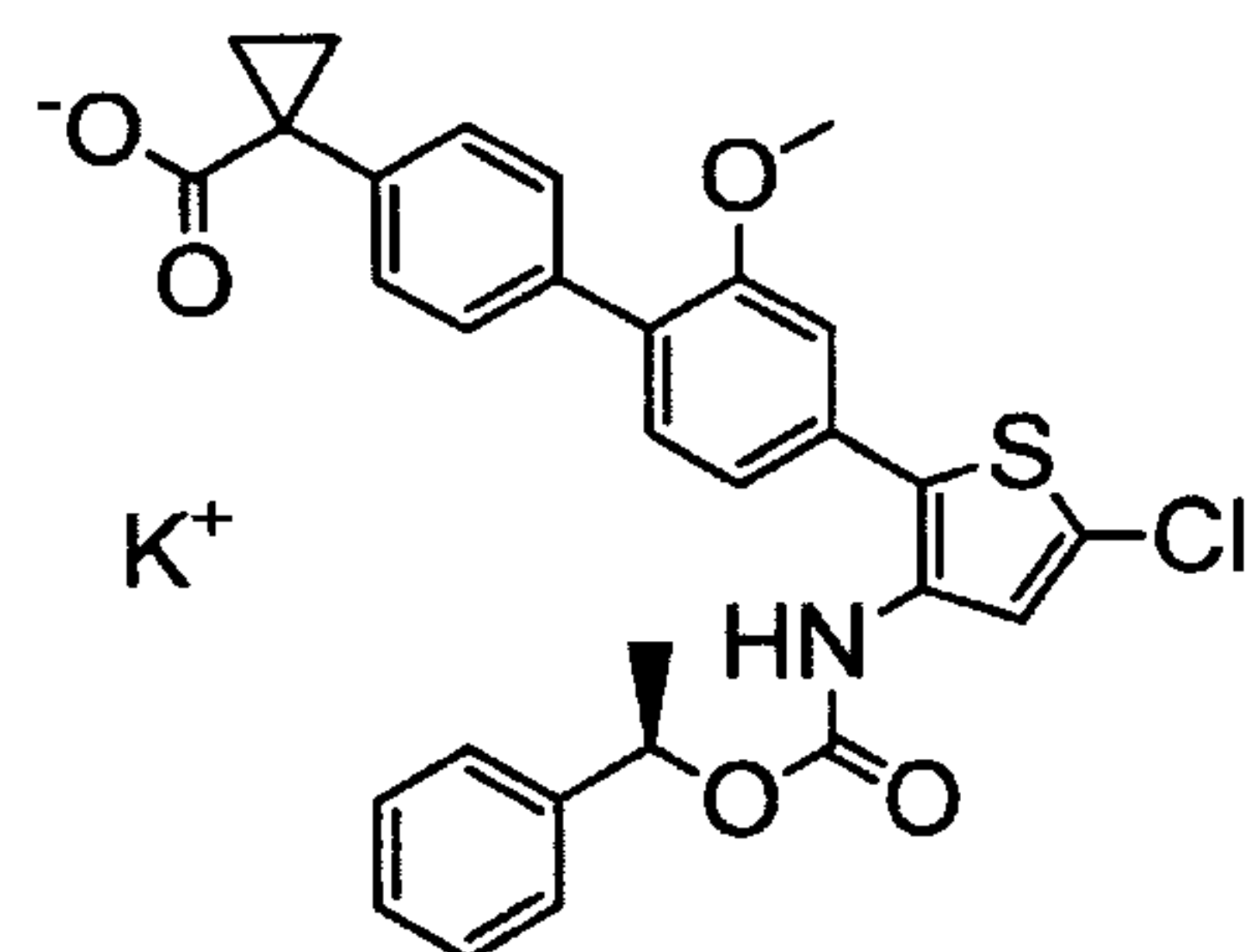
[Chem. 25]
