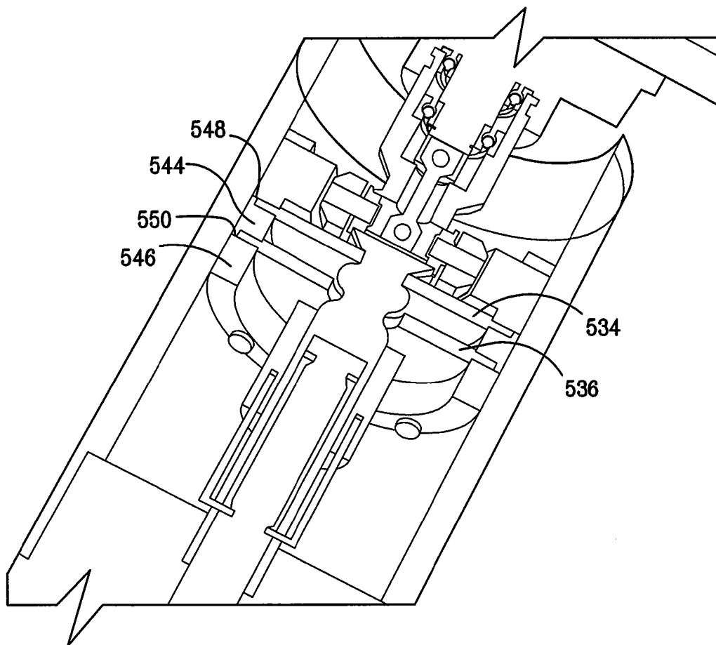
FIG. 19B
