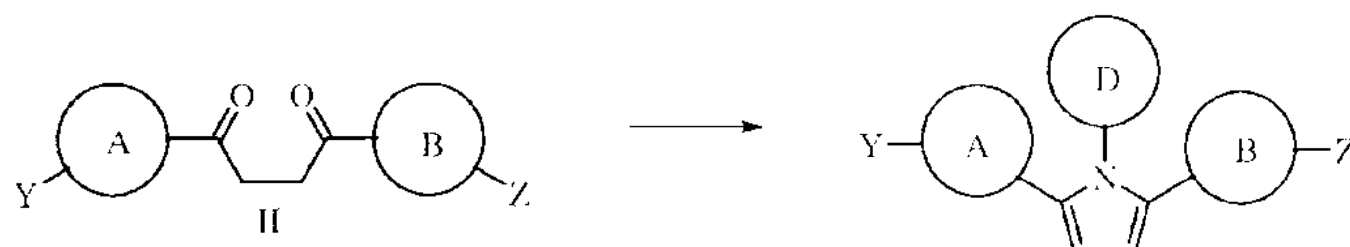
Scheme VI
