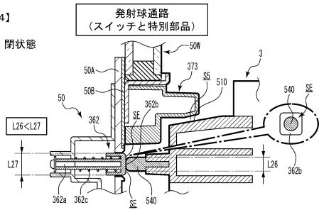
(A2) 第1開状態 (開放角度: 約2度)
