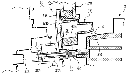
(A3) 第1開状態 (開放角度: 約5度)
