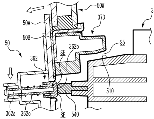
(A3) 第1開状態 (開放角度: 約5度)
