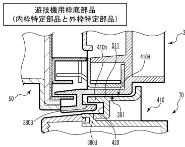
(A2) 第3開状態 (開放角度: 約2度)
