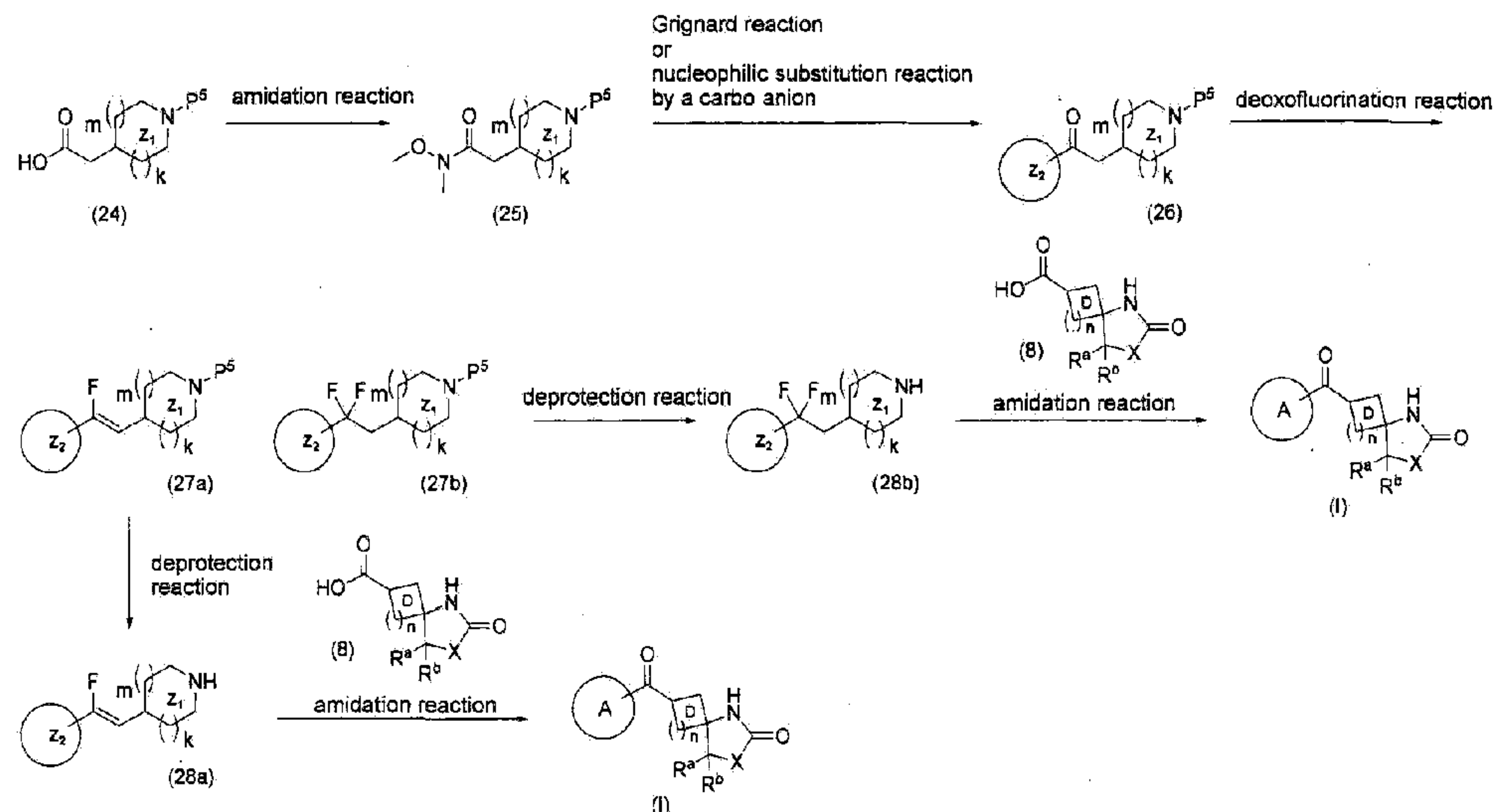
(Scheme 5)
