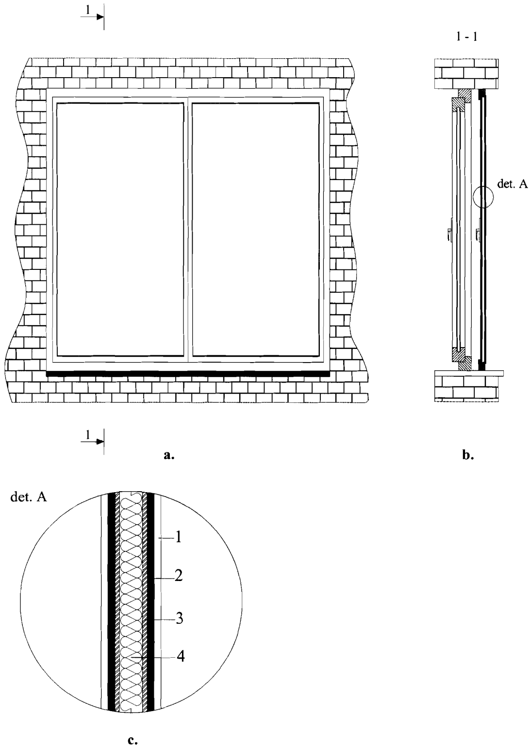
Fig. 1. Solutie termotehnica performanta tip oblon ( a. perspectiva, b. sectiune, c. detalii)
