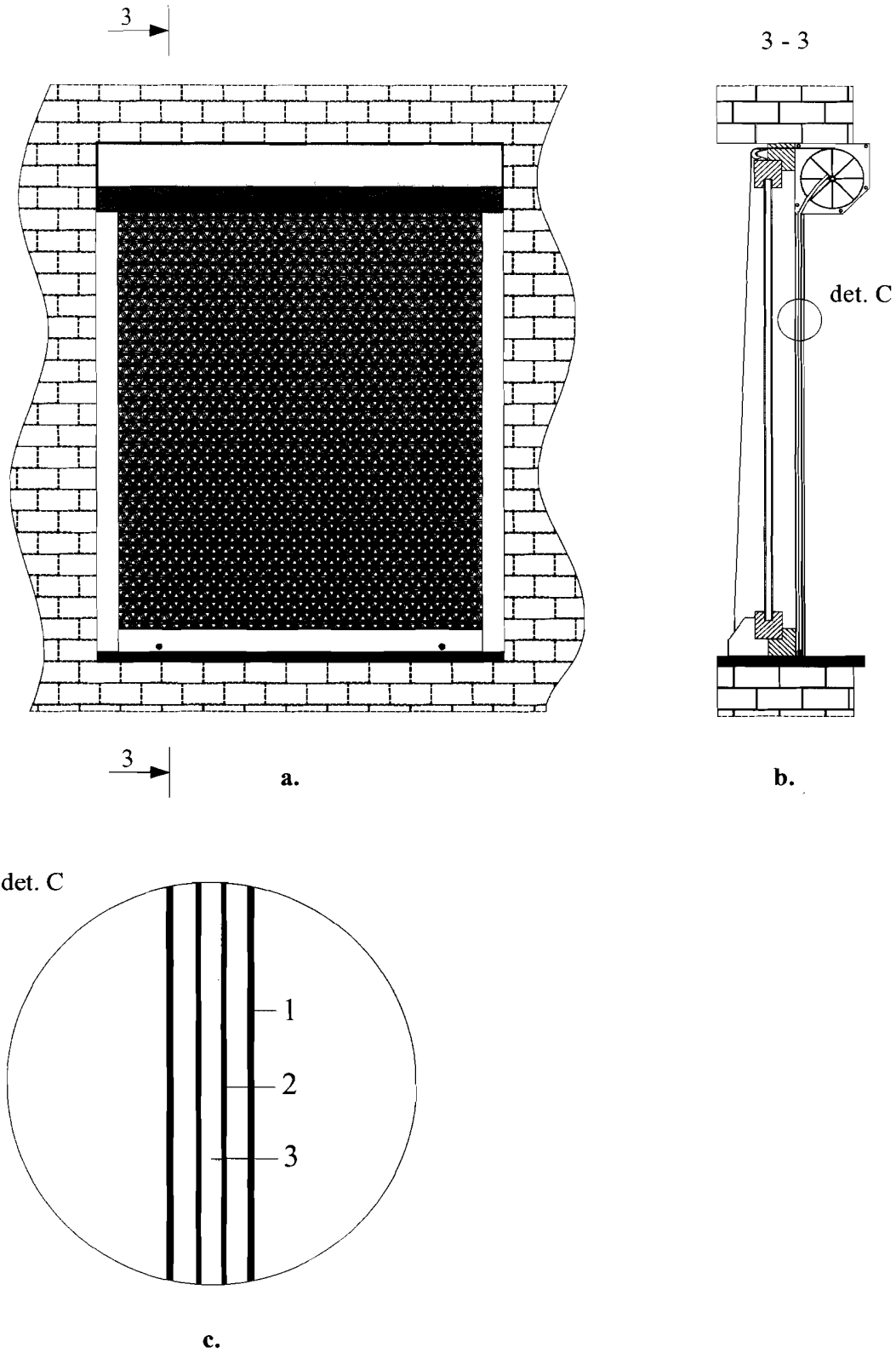
Fig. 3. Soluție termotehnică performantă tip rulou în varianta fără lamele de rigidizare (a. perspectivă, b. secțiune, c. detaliu)
