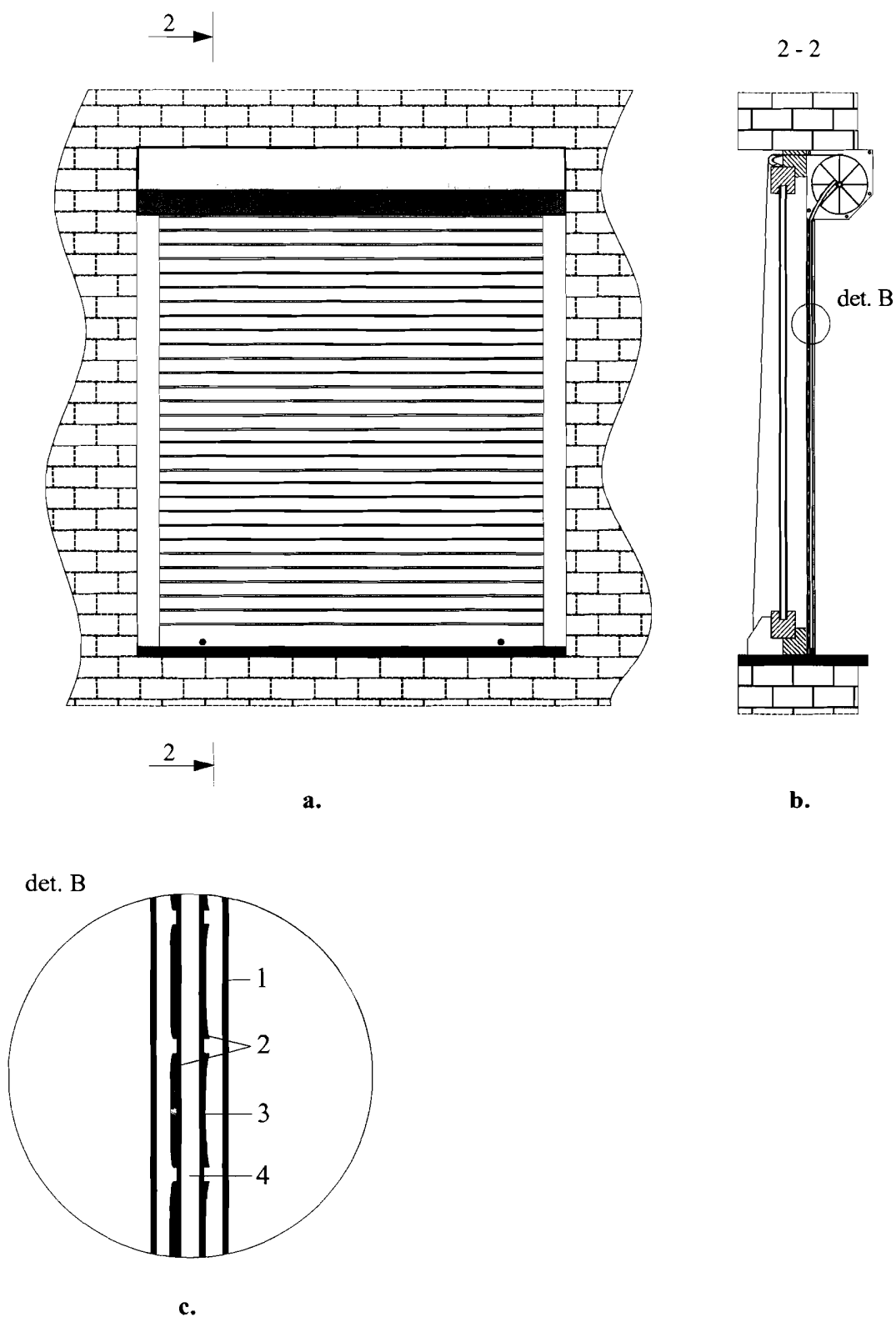
Fig. 2. Solutie termotehnica performanta tip rulou în varianta cu lamele de rigidizare (a. perspectiva, b. sectiune, c. detaliu)
