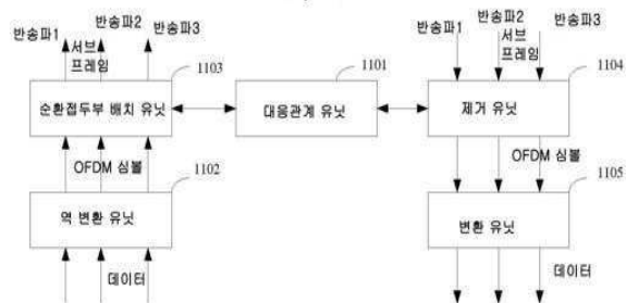
도면11
