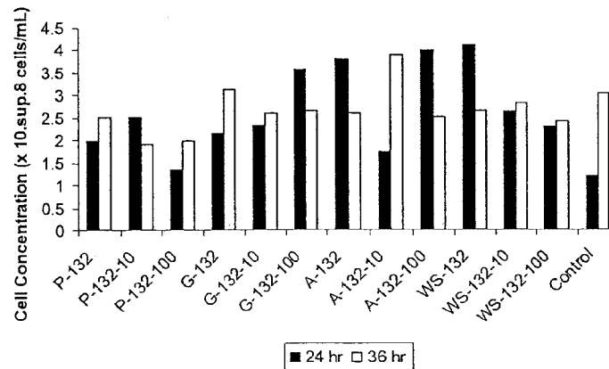
Chart 3A. Cell Concentrations for S. cerevisiae
