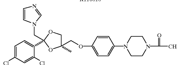
KETOCONAZOLE
