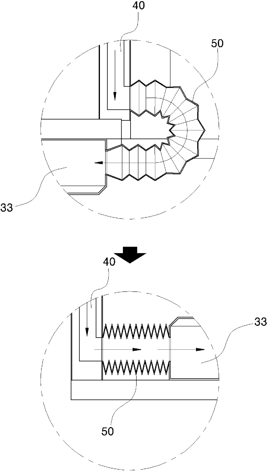
FIG.5A
