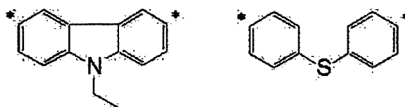
[Chem. 6]
