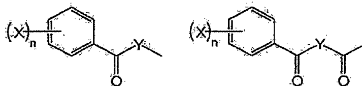
[Chem. 3]
