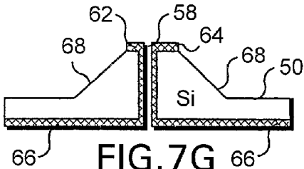
STEP 7. ANISOTROPIC ETCH
