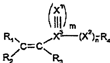
Formule I
