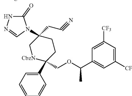
38a
