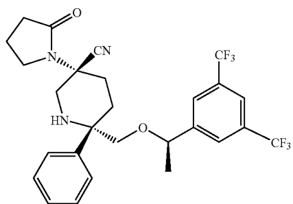
34
