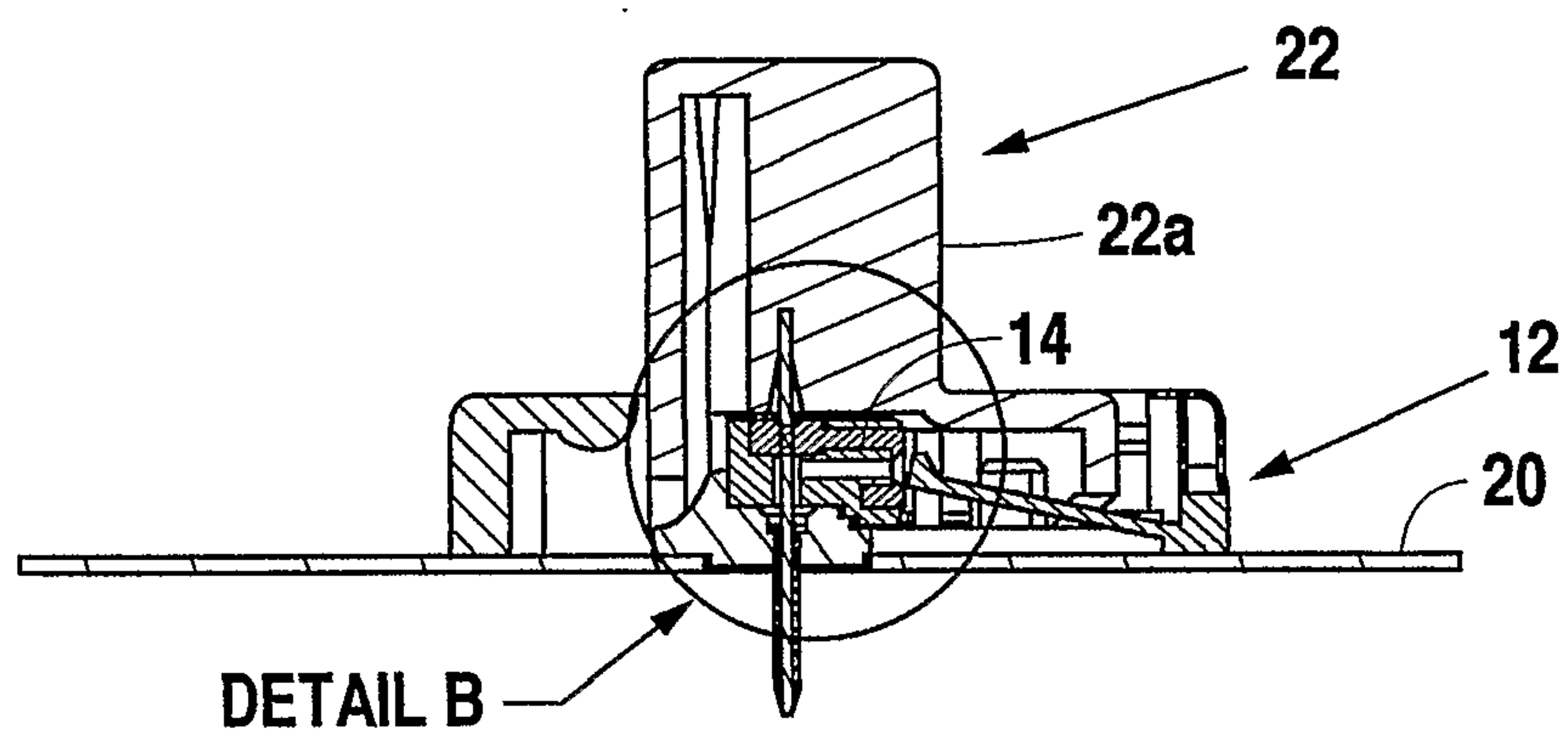
Fig. 3A ( SECTION A-A )
